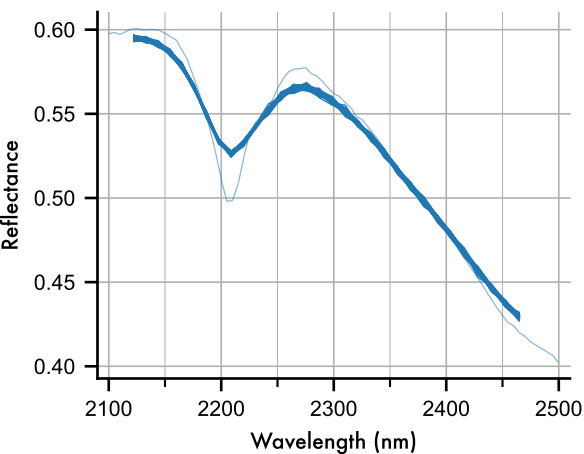
Montmorillonite
