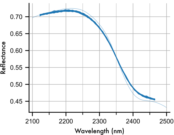
Mg-Sulphate
