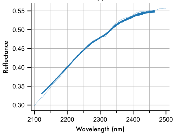
Orthopyroxene
