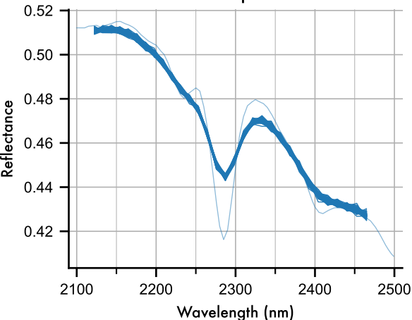
Nontronite
