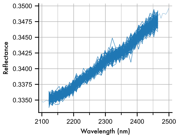
Plagioclase
