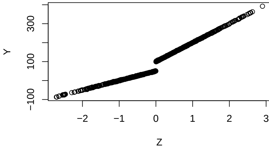
Figura 3.7.: Exemplo em que Z satisfaz o critério backdoor para medir o efeito causal de X em Y e X = \mathbb{I}(Z > 0) . Como resultado da descontinuidade da propensão de X em Z = 0 , há uma descontinuidade na regressão de Y em Z no ponto Z=0 .
