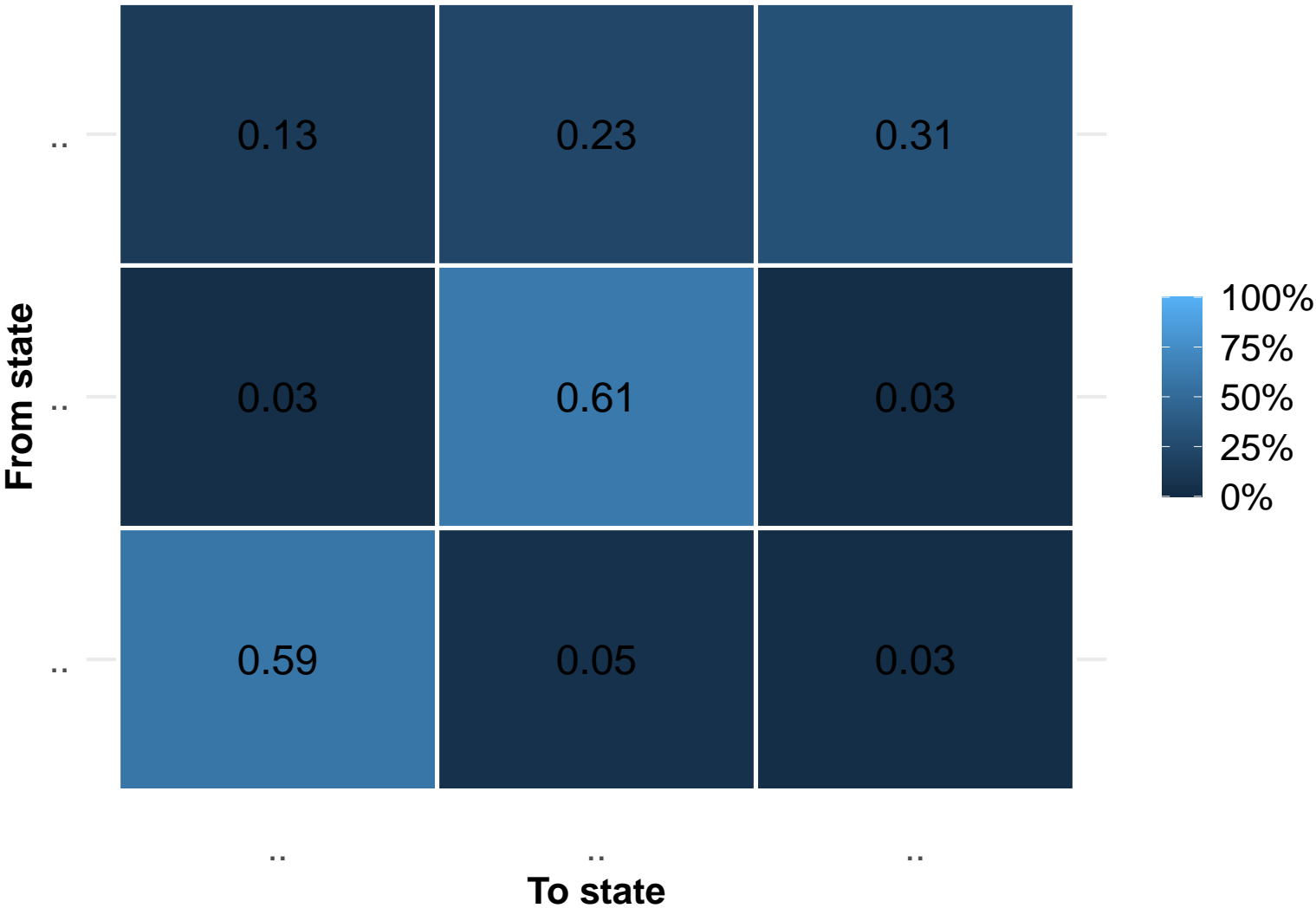
Transition probabilities (average) (K=3, mod=1)
