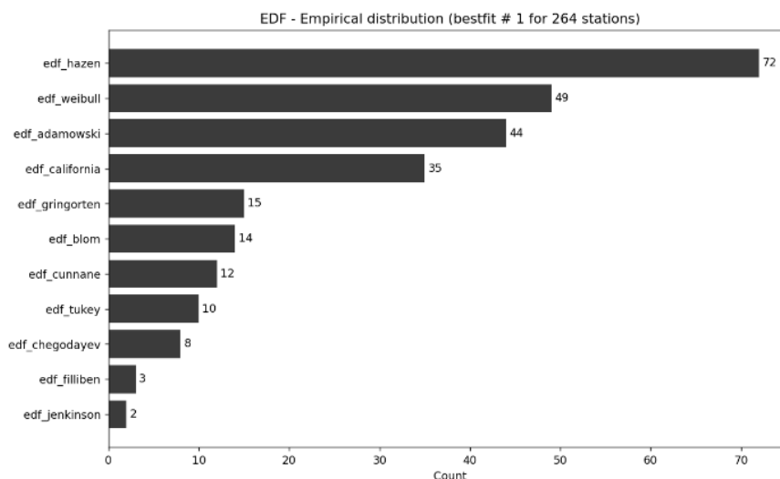
Figura 5. Clasificación de EDF con mejor ajuste global para las 264 estaciones evaluadas en Colombia.
