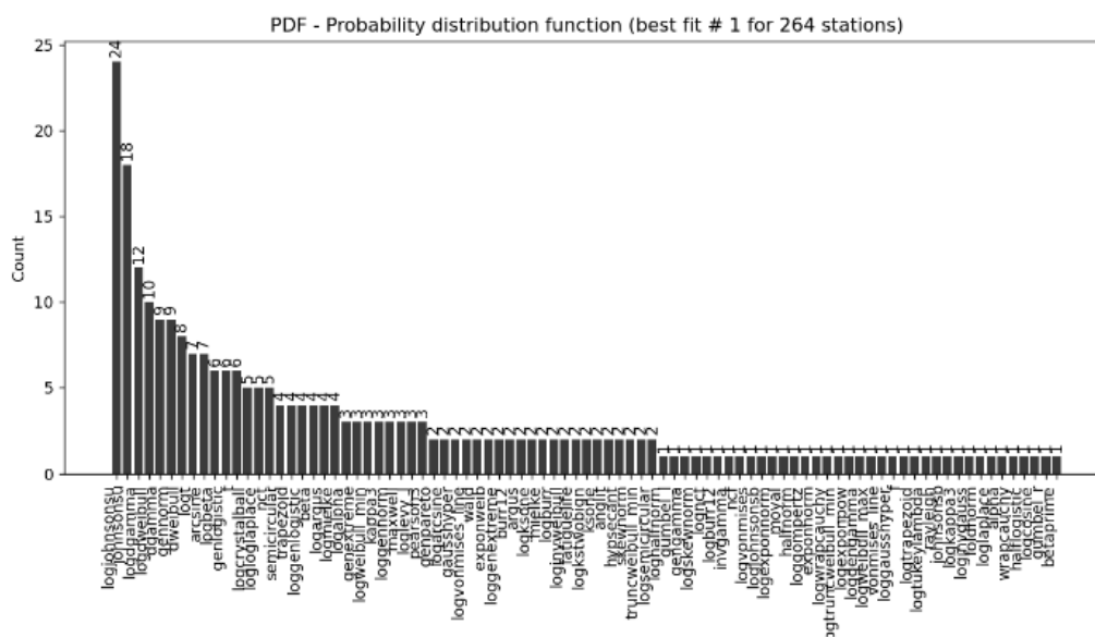
Figura 6. Clasificación de PDF con mejor ajuste global para las 264 estaciones evaluadas en Colombia.
