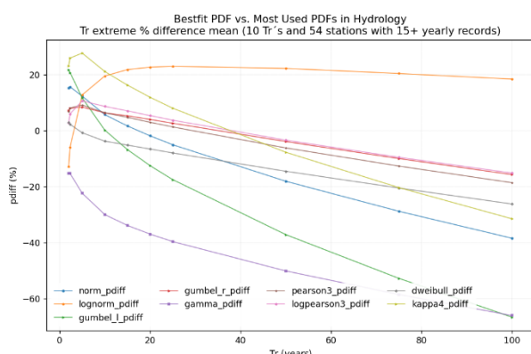
Figura 6. Diferencias porcentuales ( pdiff ) promedio entre PDF con mejor ajuste y PDF's comúnmente utilizadas en hidrología para diferentes periodos de retorno.
