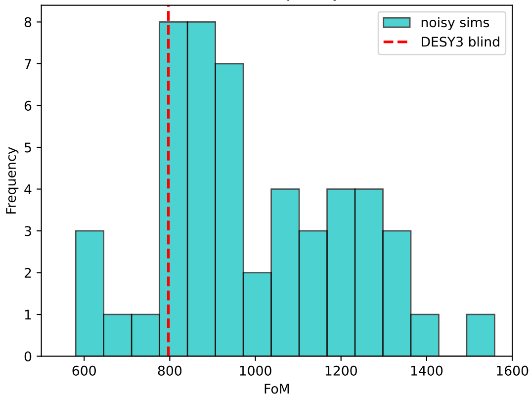
FoM values for 2pt-only chains
