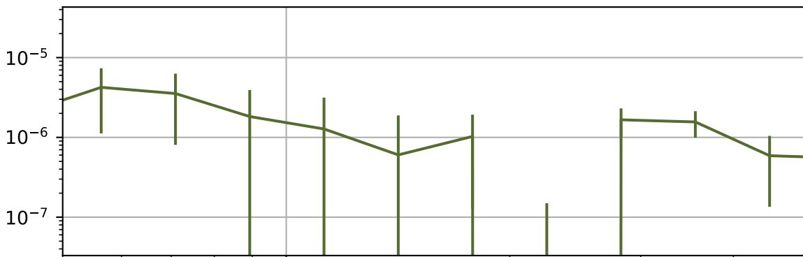
z bins 1,3
