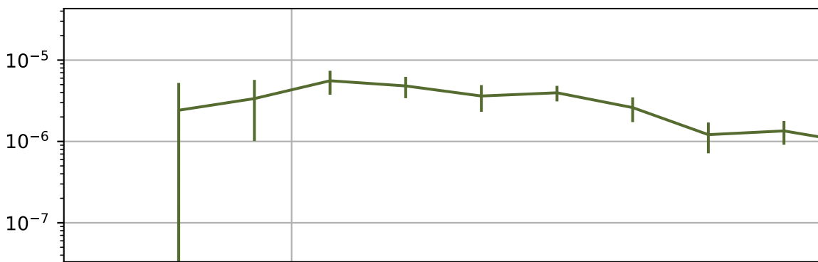
z bins 2,4
