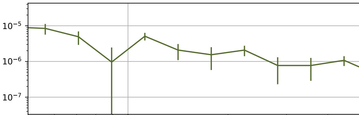
z bins 2,2
