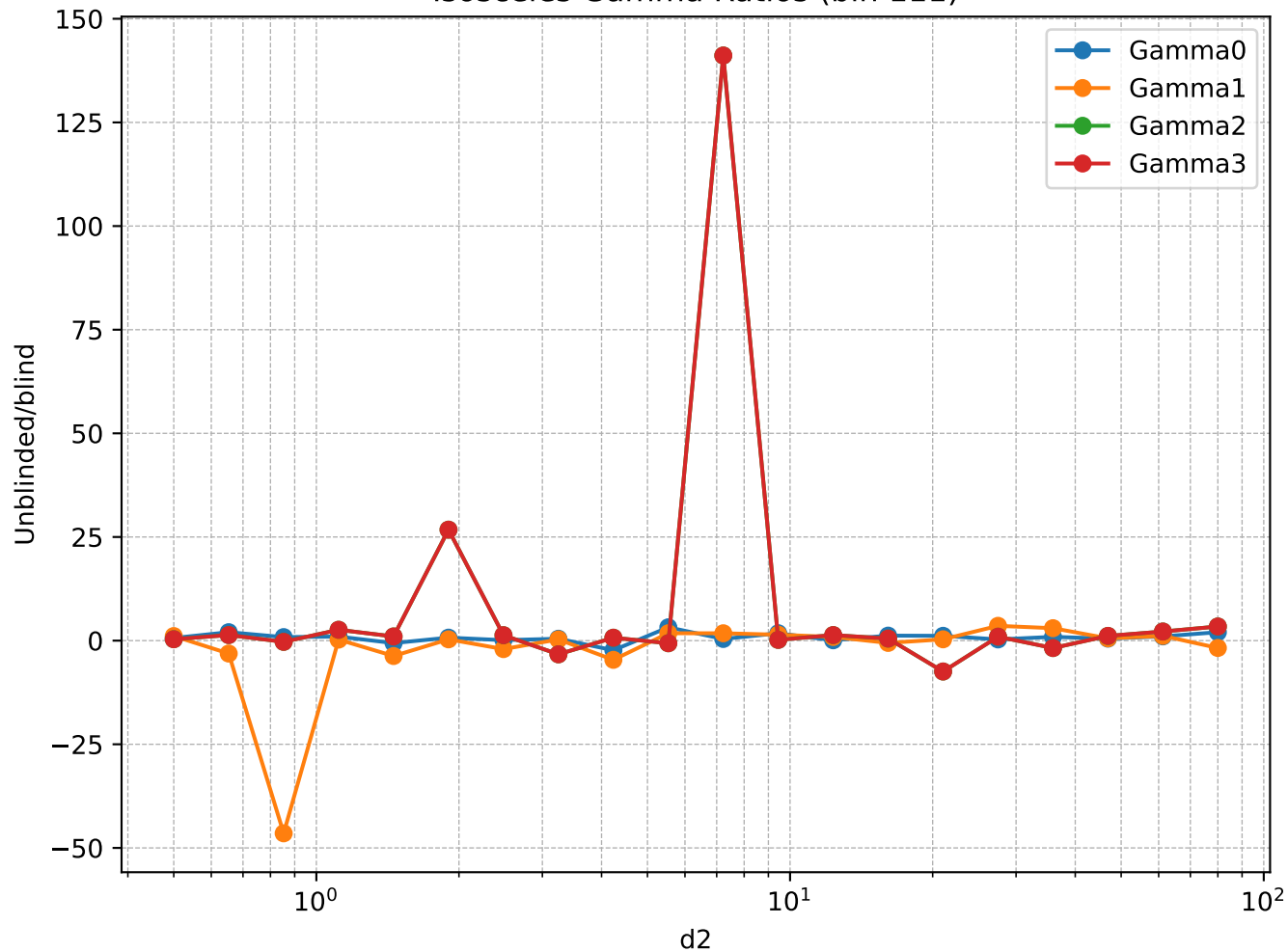
Isosceles Gamma Ratios (bin 111)
