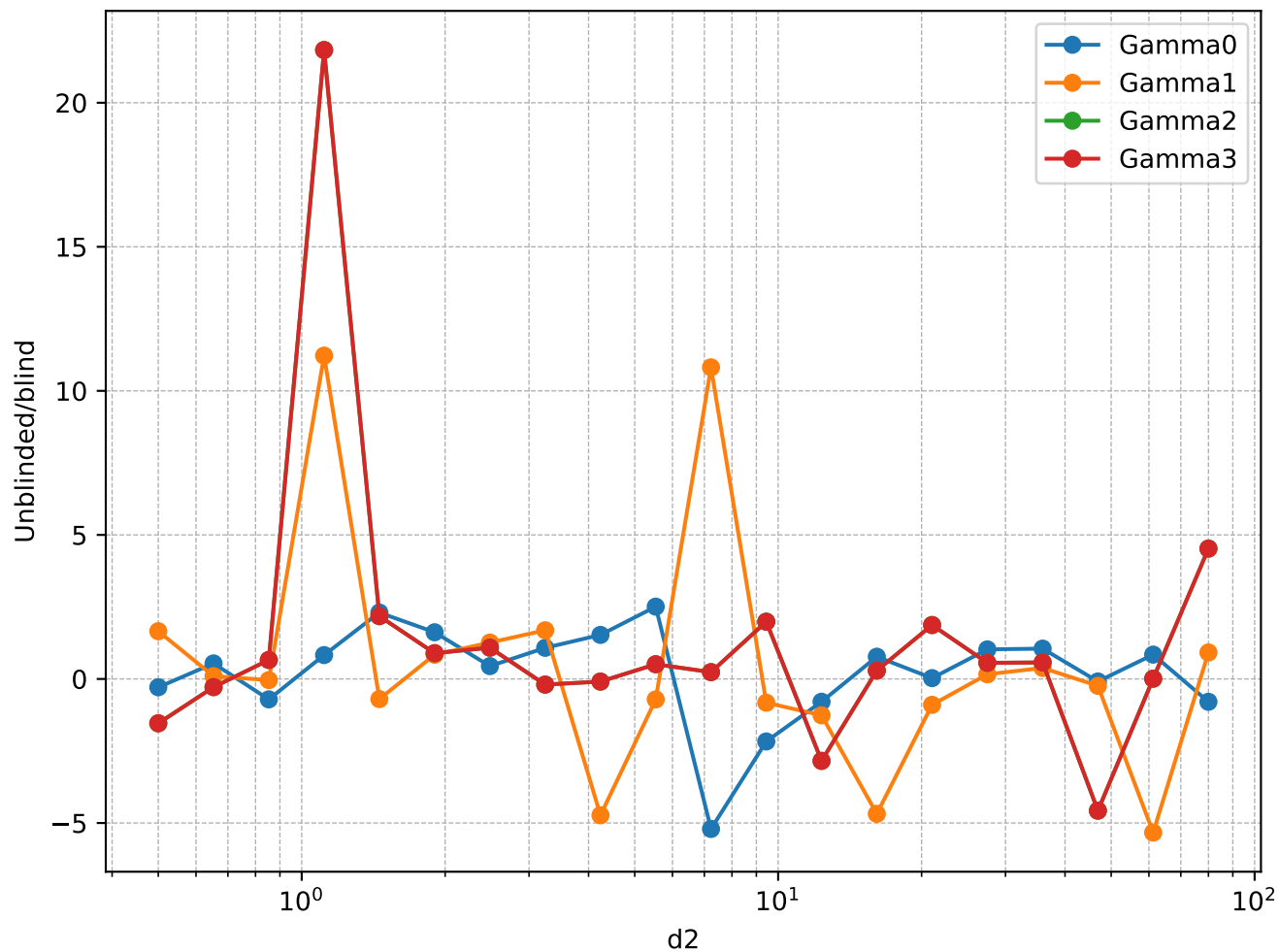
Isosceles Gamma Ratios (bin 222)
