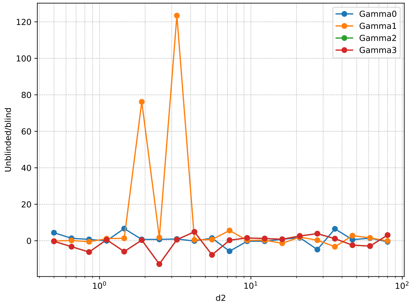
Isosceles Gamma Ratios (bin 333)
