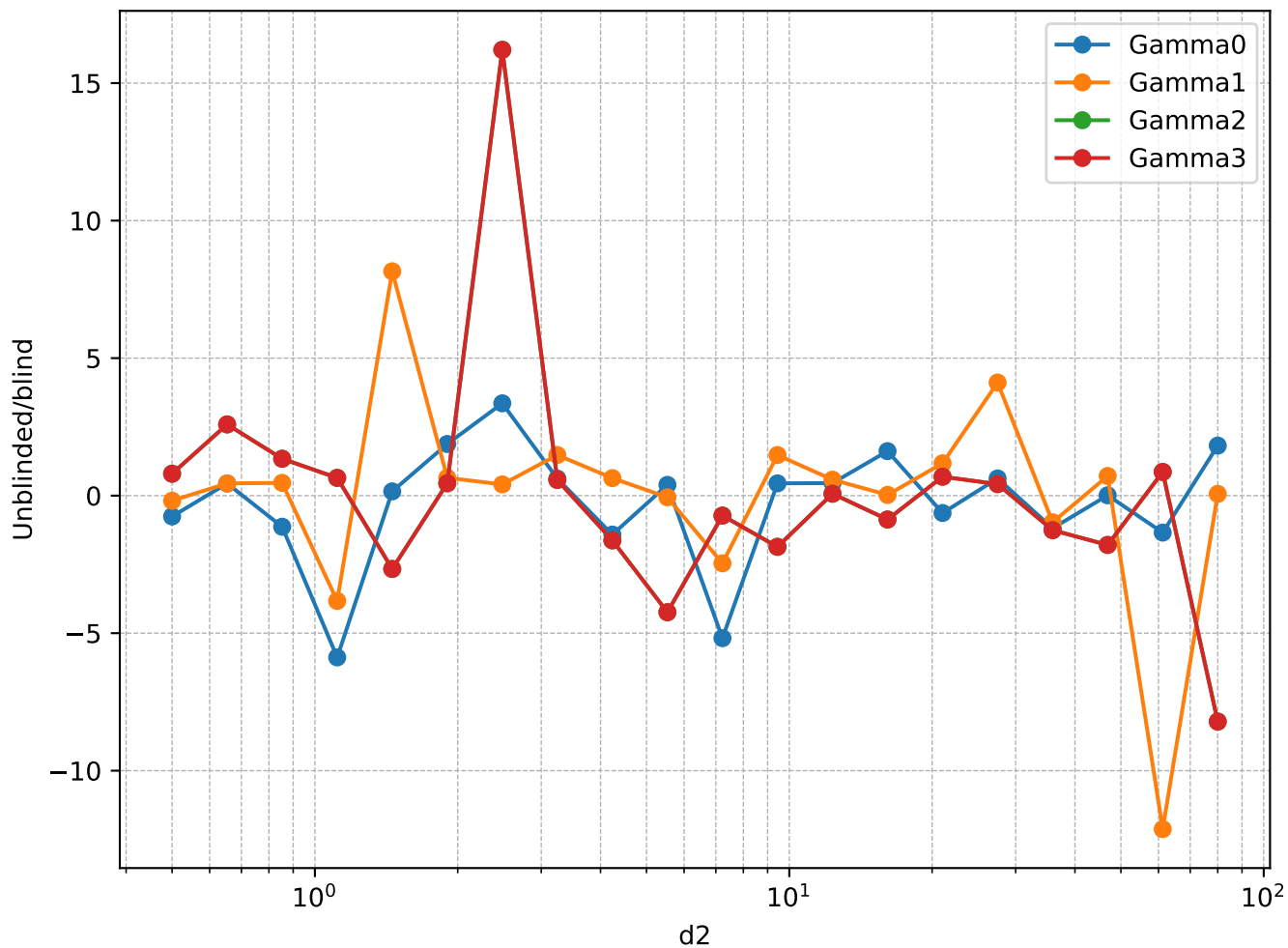
Isosceles Gamma Ratios (bin 444)
