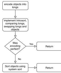
Fig. 1. HuskySort Flow
