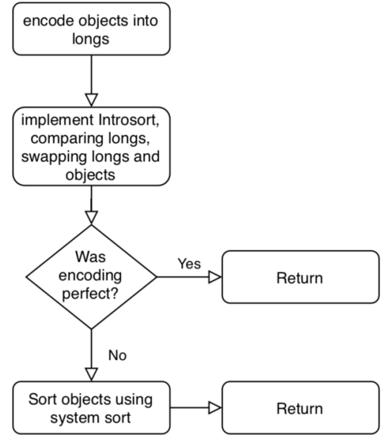
Fig. 1. Huskysort Flow
