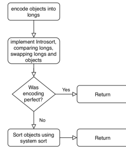
Fig. 1. Huskysort Flow
