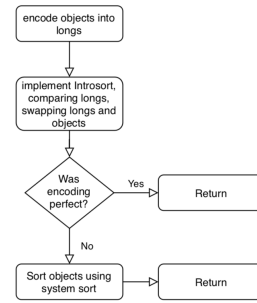
Fig. 1. Huskysort Flow
