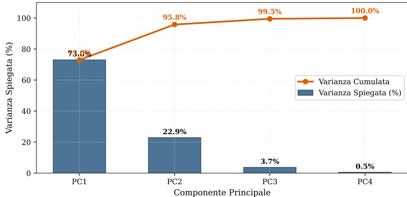
Varianza Spiegata per Componente Principale (Scree Plot)
