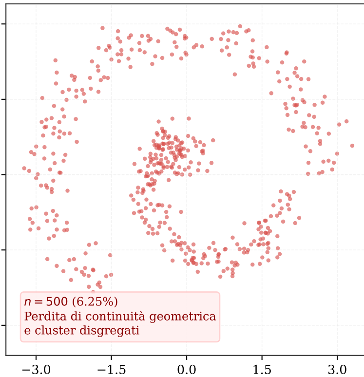
Campione Sotto-dimensionato ( n = 500 )
