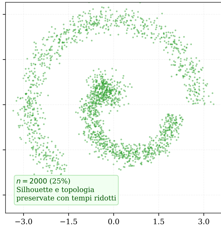
Campione Rappresentativo ( n = 2000 )
