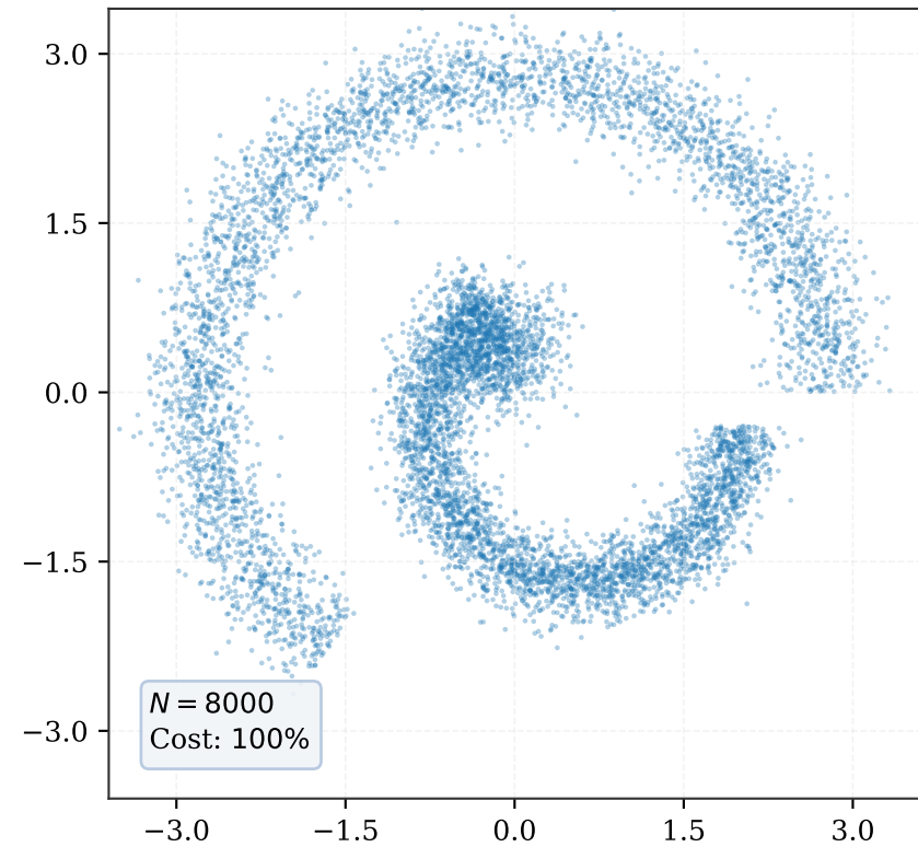
Popolazione Originaria ( N = 8000 )
