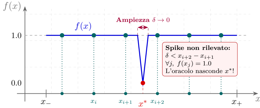
Figura 11.1: La patologia dello spike continuo: anche su un compatto [x_-, x_+] , una funzione continua può precipitare verso il minimo su una base \delta più stretta della distanza tra due campionamenti adiacenti, eludendo qualsiasi reticolo finito di nodi.
