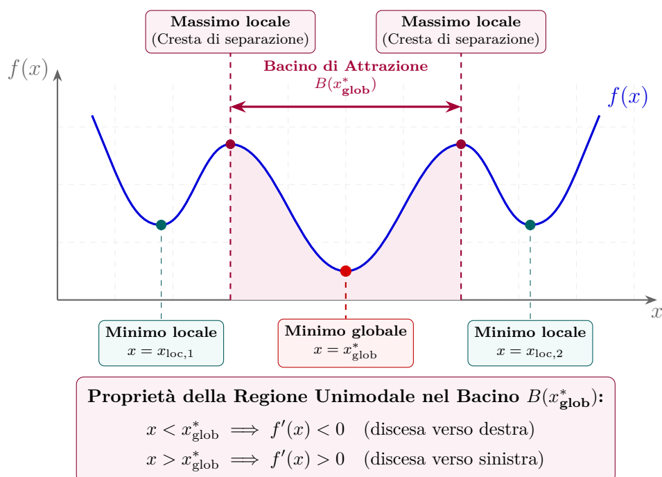
Figura 11.3: Paesaggio non convesso con molteplici minimi locali: all'interno del bacino di attrazione B(x_{\text{glob}}^*) delimitato dalle creste adiacenti la funzione è unimodale, garantendo la convergenza deterministica dei metodi locali.
