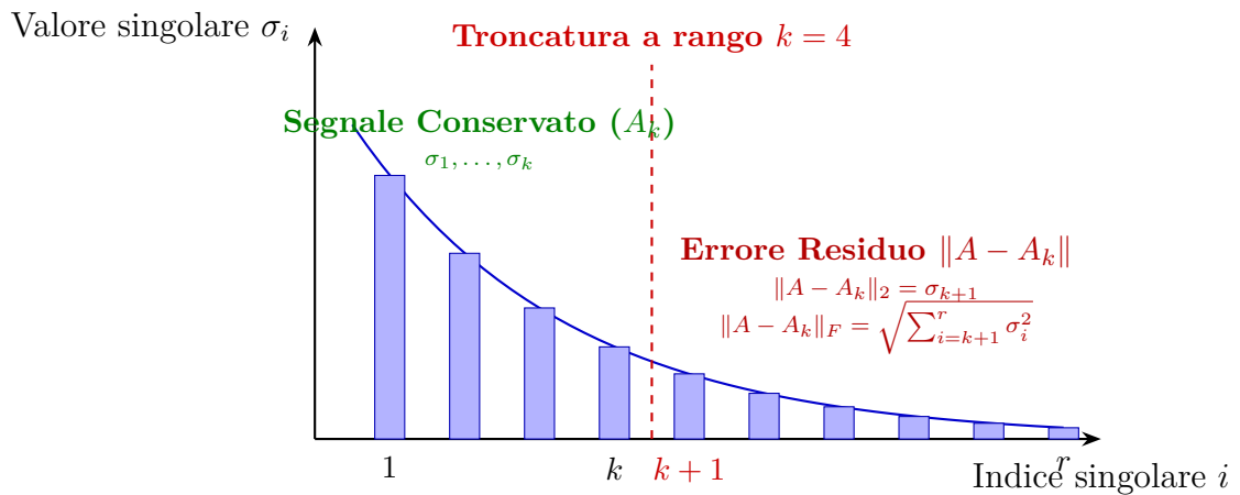
Figura 5.2: Decadimento dello spettro singolare e partizione dell'energia tra segnale conservato nell'approssimazione a rango k ( A_k ) ed errore residuo quantificato dal Teorema di Eckart-Young.
