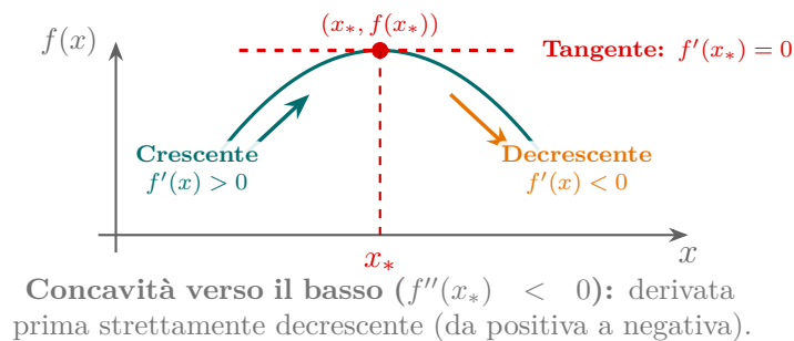
Figura 11.4: Confronto geometrico tra minimo e massimo locale sulla base del segno della derivata seconda f''(x_*) : la concavità locale determina la transizione di segno della derivata prima nell'intorno del punto stazionario.
