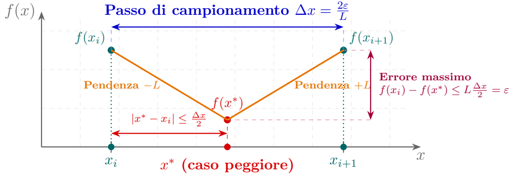
Figura 11.2: Analisi dell'errore nel caso peggiore per campionamento uniforme: se la funzione è L -Lipschitziana, nel caso peggiore il minimo x^* si colloca al punto medio \Delta x/2 , limitando l'errore di valore a L \frac{\Delta x}{2} \leq \varepsilon .
