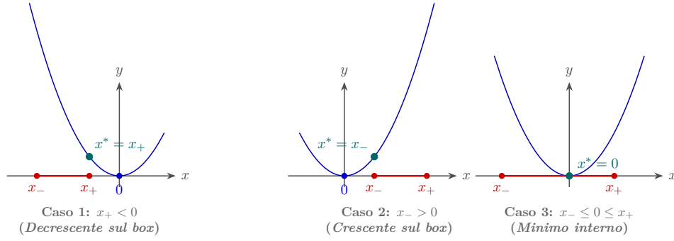
Figura 4.1: Le tre configurazioni topologiche per l'ottimizzazione quadratica omogenea vincolata su box [x_-, x_+] .
