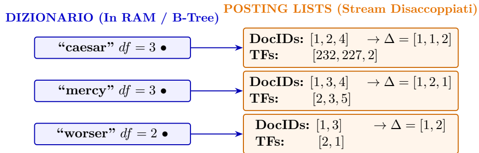
Figura 6.2: Anatomia di un indice invertito con disaccoppiamento fisico tra stream dei DocID (compressi tramite d -gaps) e stream delle frequenze tf.
