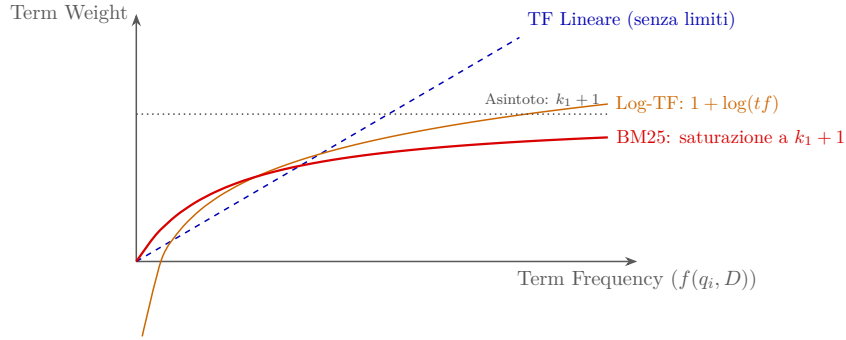
Figura 5.2: Confronto qualitativo tra crescita del TF lineare, TF logaritmico e saturazione asintotica in BM25.
