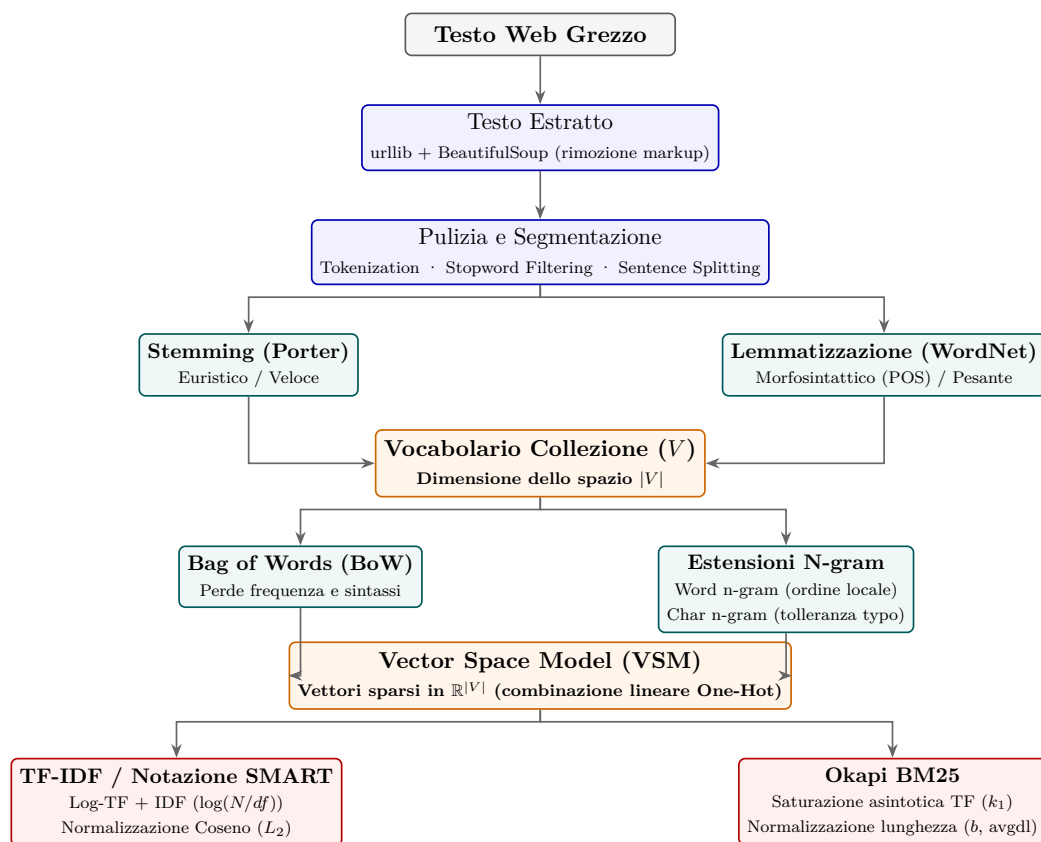
Figura 5.3: Mappa concettuale integrata della pipeline di IR: dall'acquisizione del testo ai modelli di recupero vettoriali e probabilistici.
