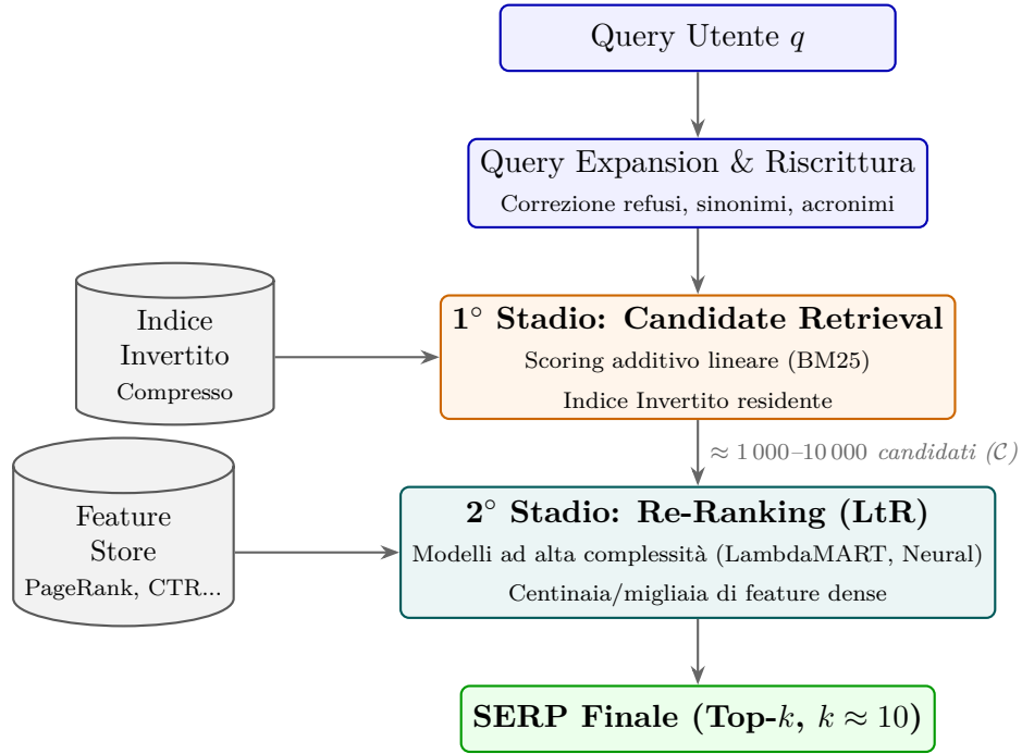
Figura 6.1: Architettura del paradigma di retrieval a due stadi: filtraggio massivo ad alta efficienza (primo stadio) e riordinamento semantico ad alta accuratezza (secondo stadio).
