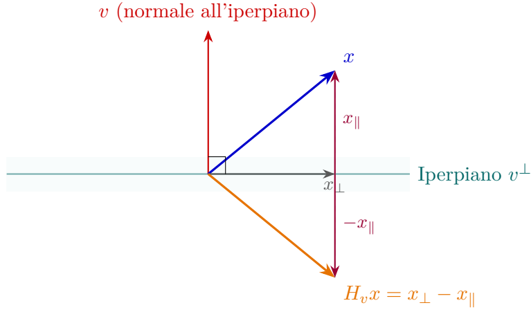
Figura 6.2: Interpretazione geometrica dell'azione del riflettore di Householder: riflessione speculare rispetto all'iperpiano v^\perp .
