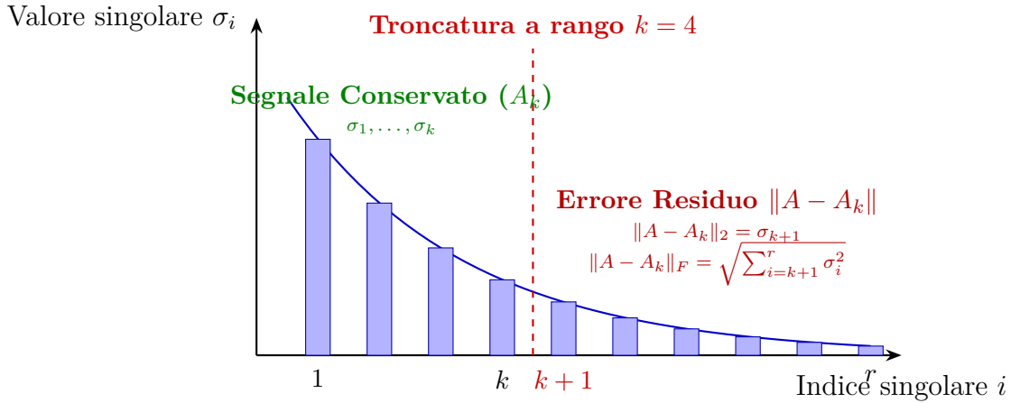
Figura 5.2: Decadimento dello spettro singolare e partizione dell'energia tra segnale conservato nell'approssimazione a rango k ( A_k ) ed errore residuo quantificato dal Teorema di Eckart-Young.
