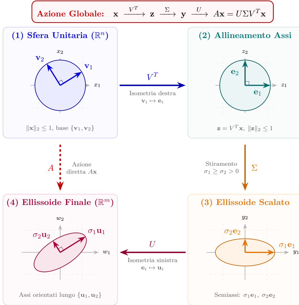
Figura 5.3: Interpretazione geometrica dell'azione di una matrice A = U\Sigma V^T sulla sfera unitaria euclidea rappresentata a quattro quadranti: (1) Sfera originaria con i vettori singolari destri \mathbf{v}_i ; (2) Isometria V^T che allinea le direzioni \mathbf{v}_i con la base canonica \mathbf{e}_i ; (3) Deformazione assi-simmetrica \Sigma che genera un ellissoide con semiassi \sigma_i ; (4) Isometria finale U che orienta i semiassi dell'ellissoide lungo i vettori singolari sinistri \mathbf{u}_i .
