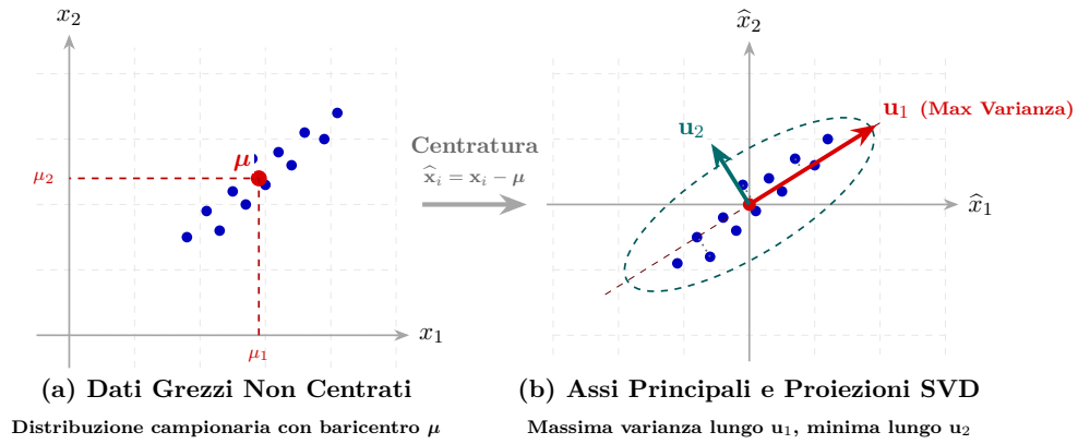
Figura 5.4: Interpretazione geometrica dell'Analisi delle Componenti Principali (PCA) via SVD: (a) Distribuzione iniziale con baricentro \mu ; (b) Dati centrati con le direzioni principali \mathbf{u}_1 (massima varianza) e \mathbf{u}_2 ortogonale ricavate dalla SVD della matrice centrata \hat{A} = U\Sigma V^T , con proiezioni ortogonali sul sottospazio ottimo.
