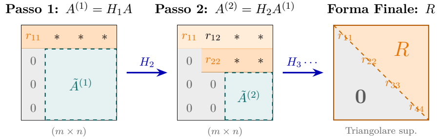
Figura 6.3: Progressione iterativa dell'annullamento sotto-diagonale tramite l'algoritmo di Householder QR.
