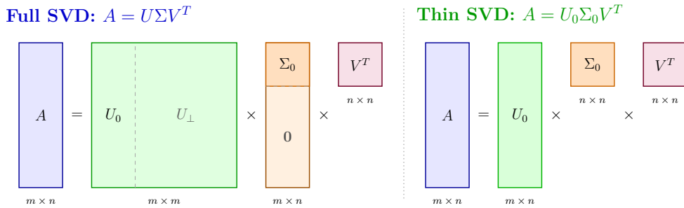
Figura 5.1: Confronto geometrico e dimensionale tra Full SVD ed Economy (Thin) SVD per matrici ad asse verticale ( m \geq n ). Nella Thin SVD il blocco inferiore nullo di \Sigma e le colonne superflue U_\perp vengono omesse.
