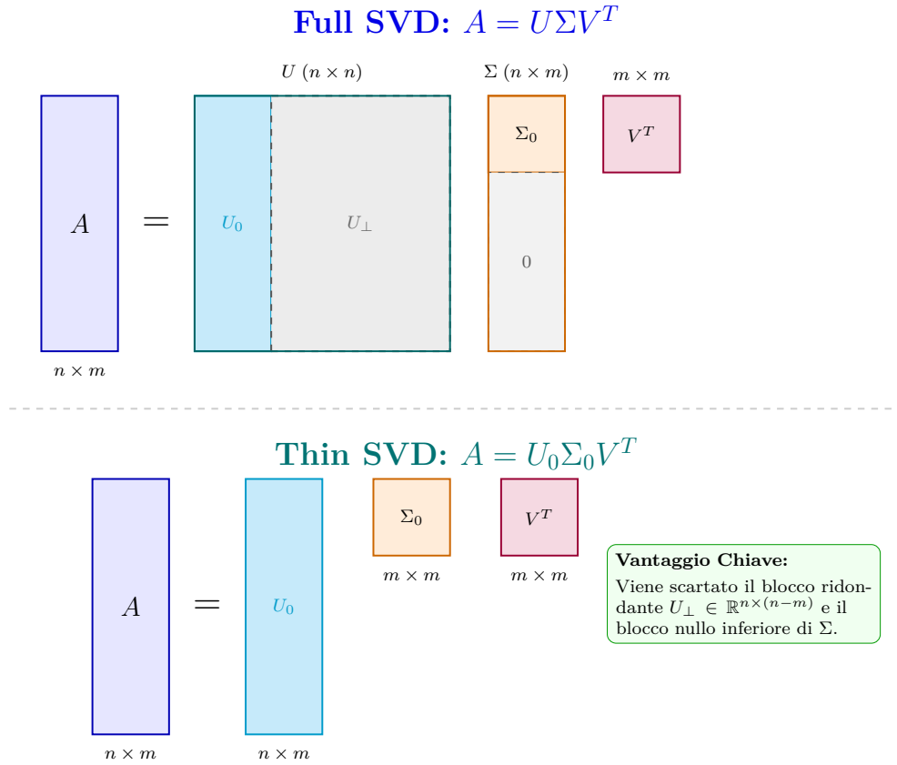
Figura 4.1: Confronto geometrico e strutturale a blocchi tra Full SVD e Thin SVD per una matrice alta e stretta ( n > m ).
