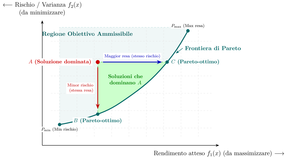
Figura 8.1: Rappresentazione geometrica della Frontiera di Pareto nel problema di selezione di portafoglio di Markowitz.
