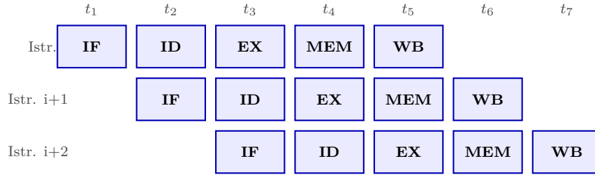
Figura 3.1: Sovrapposizione degli stadi della pipeline a 5 stadi su istruzioni consecutive.
