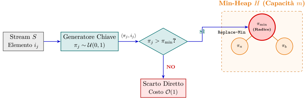
Figura 7.2: Schema funzionale del Priority Sampling su stream mediante Min-Heap di capienza fissa m .
