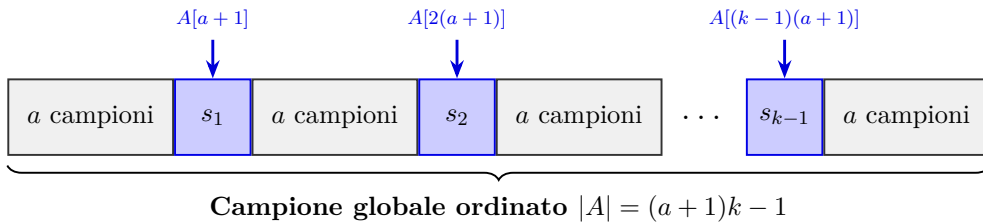
Figura 6.2: Topologia dell'array ausiliario ordinato A : tra ciascuna coppia di pivot contigui cadono esattamente a campioni intermedi.
