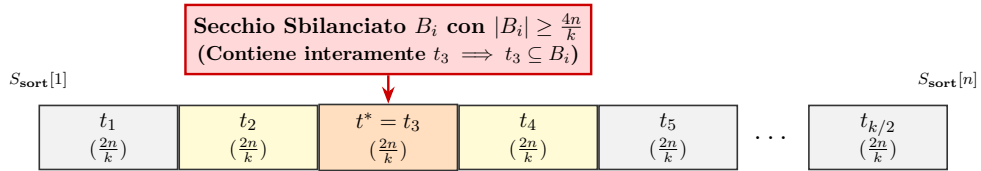
Figura 6.3: Costruzione geometrica di contenimento: un secchio B_i di taglia \geq 4n/k copre interamente almeno un segmento logico t^* \subset S_{\text{sort}} di ampiezza 2n/k .
