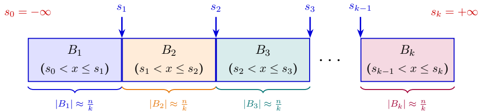
Figura 6.1: Partizionamento dell'universo delle chiavi in k secchi disgiunti mediante k - 1 pivot ordinati e due sentinelle concettuali.
