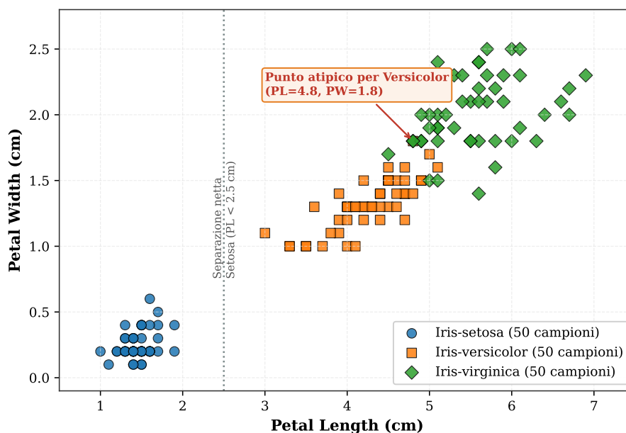
Figura 3.1: Scatter plot bivariati sul dataset Iris: confronto tra la separabilità generata da sepal e petalo.
