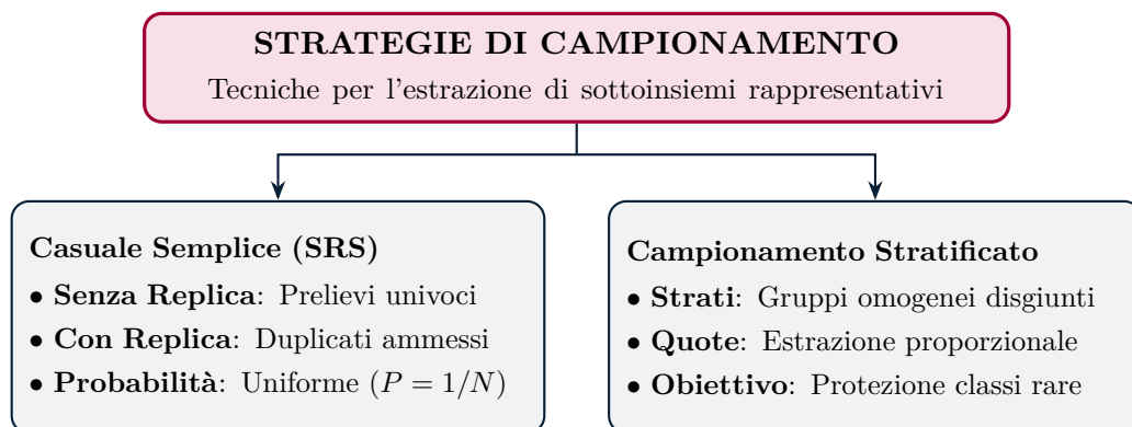
Figura 4.3: Albero delle strategie di campionamento nel data mining.
