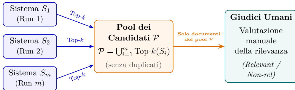
Figura 2.2: Processo di Pooling per la selezione controllata dei documenti da annotare.
