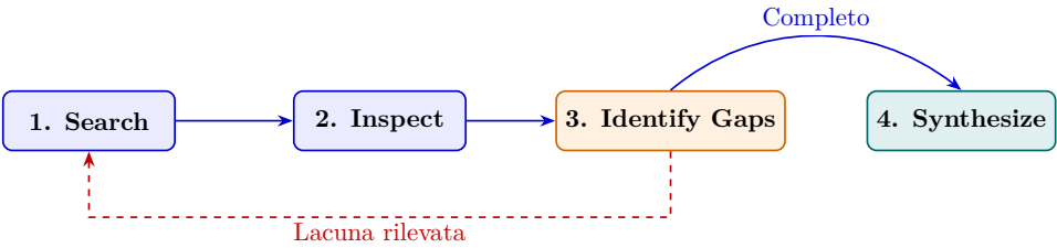
Figura 1.1: Ciclo a retroazione adattivo ( Adaptive Feedback Loop ) dell'Agentic Search.
