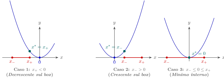
Figura 5.1: Le tre configurazioni topologiche per l'ottimizzazione quadratica omogenea vincolata su box [x_-, x_+] .
