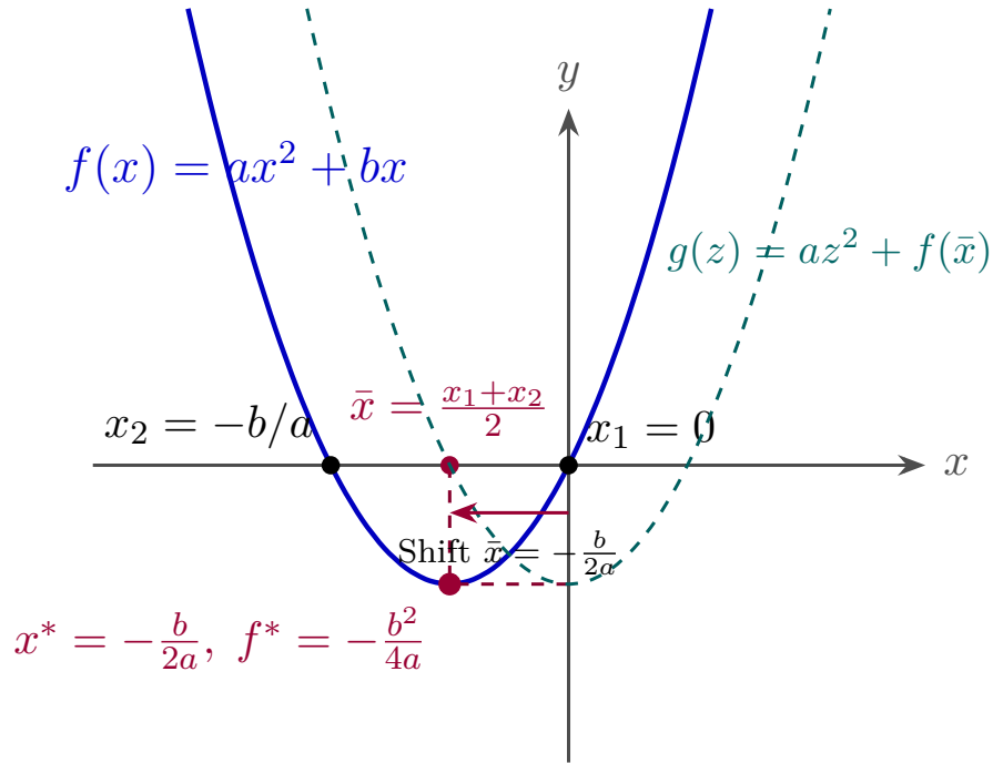
Figura 5.2: Visualizzazione geometrica del cambio di coordinate per la parabola non omogenea: il vertice x^* si colloca esattamente a metà strada tra le due radici x_1 e x_2 .
