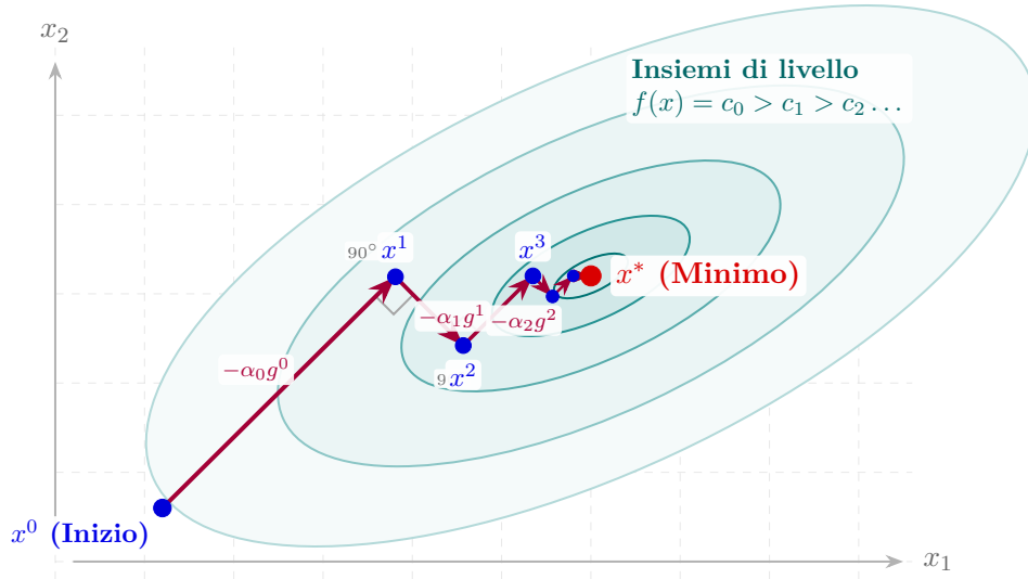
Figura 7.2: Traiettorie a zig-zag del metodo GMQ su insiemi di livello ellittici: la scelta analitica del passo ottimale impone la perfetta ortogonalità tra direzioni successive ( \langle g^{k+1}, g^k \rangle = 0 ), costringendo le iterate a compiere svolte ad angolo retto esatto ( 90^\circ ).
