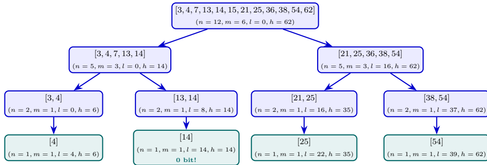
Figura 1.4: Albero di decomposizione dicotomica del Binary Interpolative Coding.
