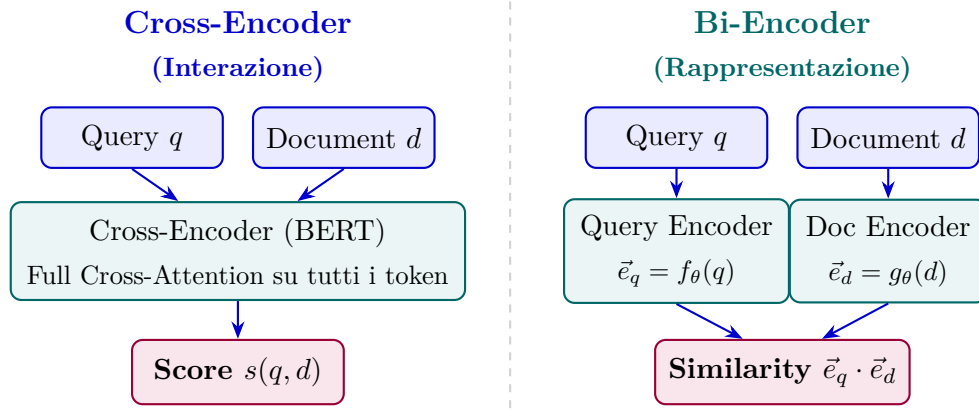
Figura 1.6: Confronto strutturale tra Cross-Encoder (Interazione) e Bi-Encoder (Rappresentazione).
