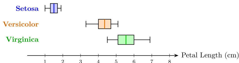
Figura 2.2: Esempio di Box Plot Condizionale: distribuzione dell'attributo Petal Length condizionata alla specie di fiore nel dataset Iris.
