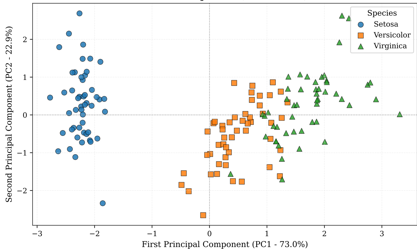
2D PCA Projection (Iris Dataset)
