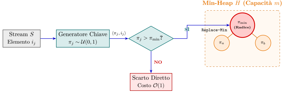
Figura 7.2: Schema funzionale del Priority Sampling su stream mediante Min-Heap di capienza fissa m .
