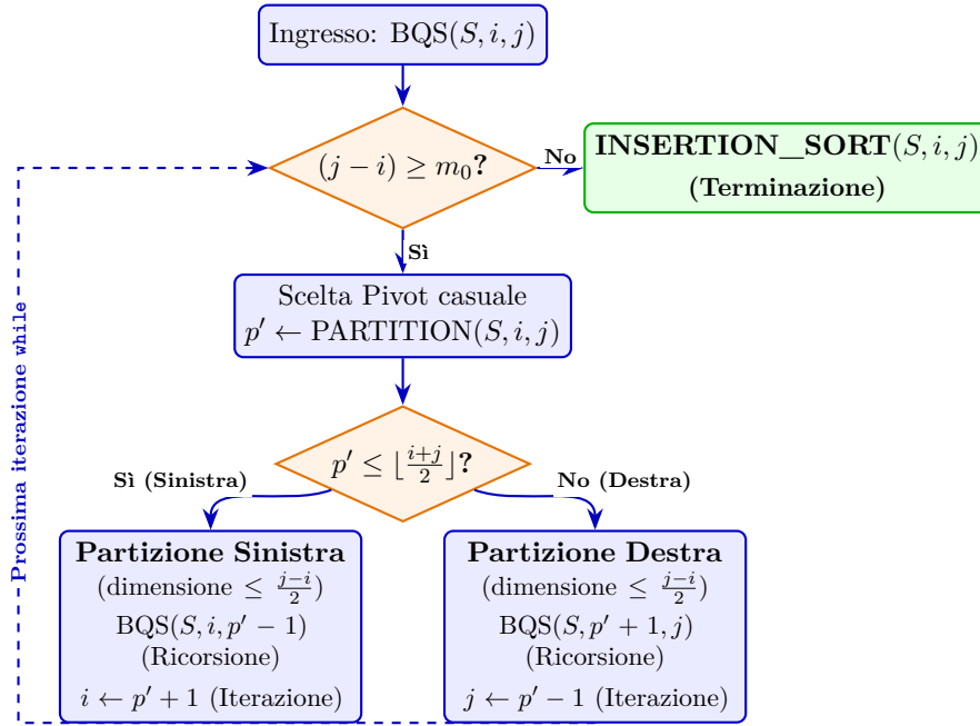
Figura 4.4: Diagramma di controllo del Bounded Quicksort (BQS). La chiamata ricorsiva viene lanciata rigidamente sulla metà di dimensione minore ( \leq (j - i)/2 ), mentre la partizione più grande viene elaborata mediante iterazione continua nel ciclo while . I blocchi inferiori a m_0 sono ordinati direttamente da Insertion Sort.
