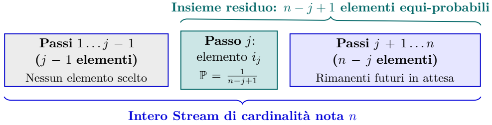
Figura 7.1: Partizione dello spazio dello stream al passo generico j per il campionamento a singolo elemento ( m = 1 ).
