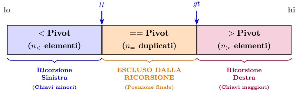
Figura 5.3: Topologia delle tre regioni del partizionamento a 3 vie ( Dutch National Flag ) e puntatori operativi lt e gt .
