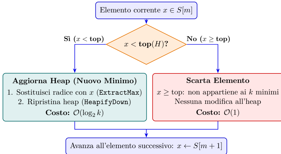
Figura 5.1: Flusso di elaborazione con Max-Heap di dimensione limitata k . Gli elementi che non migliorano i k minimi correnti vengono scartati in tempo costante \mathcal{O}(1) .
