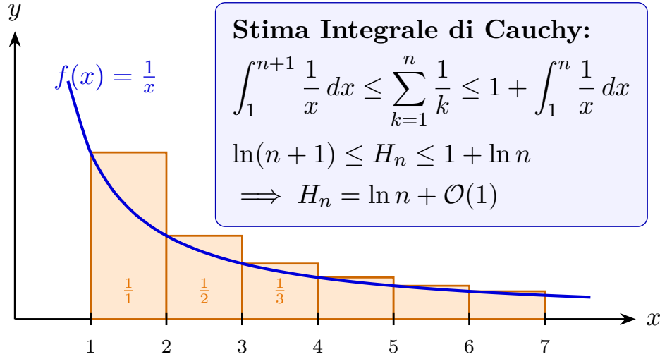
Figura 5.4: Approssimazione integrale della serie armonica H_n = \sum_{k=1}^n \frac{1}{k} \approx \ln n . L'area dei rettangoli maggiore l'integrale della funzione iperbolica f(x) = \frac{1}{x} .
