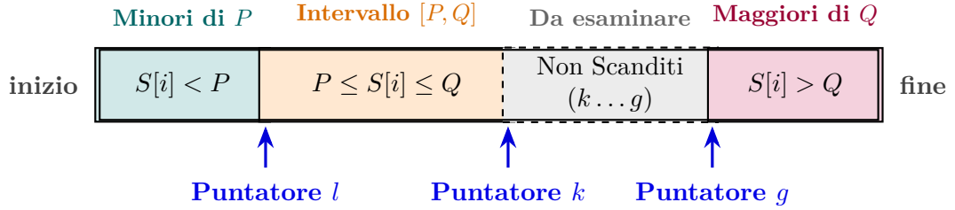
Figura 4.3: Schema del partizionamento nel Dual-Pivot Quicksort di Yaroslavskiy. L'array è partizionato nelle quattro regioni dinamiche: elementi < P , elementi compresi tra P e Q , elementi non ancora esaminati tra k e g , ed elementi > Q .
