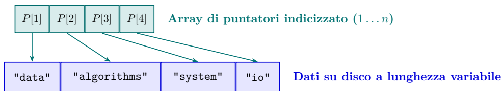
Figura 6.4: Mappatura di record a lunghezza variabile tramite array contiguo di puntatori indicizzato.
