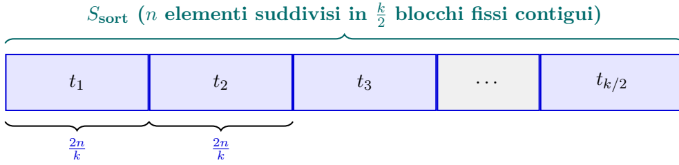
Figura 6.3: Partizione teorica di S_{\text{sort}} in \frac{k}{2} blocchi fissi t_j di cardinalità \frac{2n}{k} .
