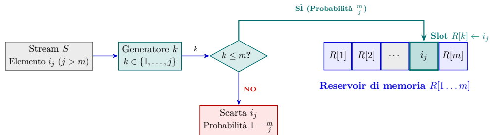
Figura 7.3: Flusso operativo di inserimento e sostituzione del Reservoir Sampling (Algoritmo R).
