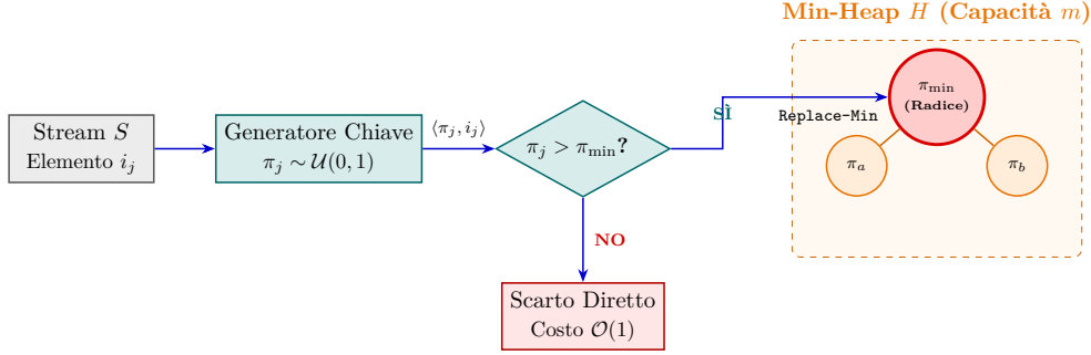
Figura 8.2: Schema funzionale del Priority Sampling su stream mediante Min-Heap di capienza fissa m .
