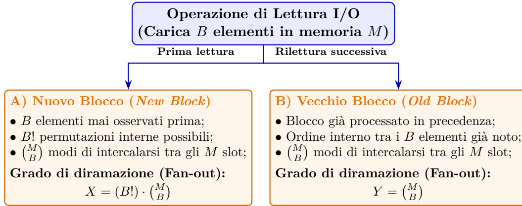
Figura 5.2: Fattori di diramazione ( fan-out ) nell'albero di decisione di I/O nel modello a due livelli: la lettura di un nuovo blocco apporta informazione d'ordine interno ( B! ) e di intercalamento ( \binom{M}{B} ); la riletture di un vecchio blocco apporta esclusivamente informazione di intercalamento.
