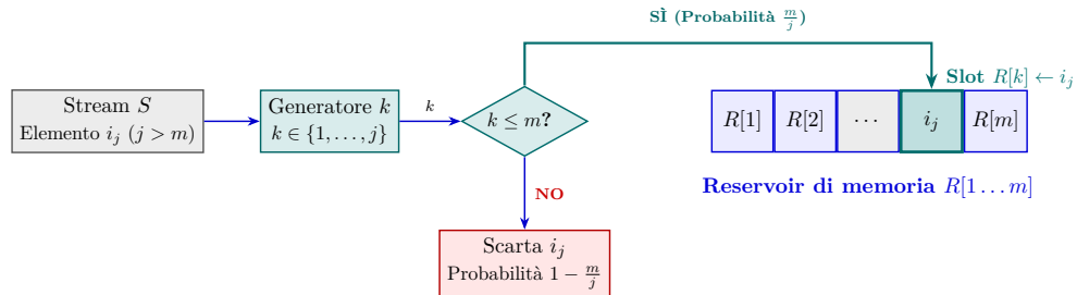
Figura 8.3: Flusso operativo di inserimento e sostituzione del Reservoir Sampling (Algoritmo R).
