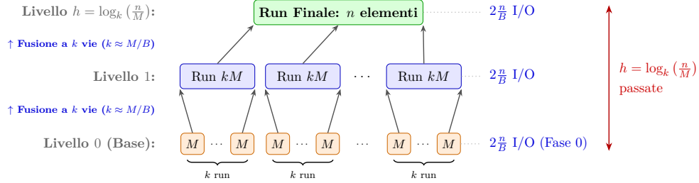
Figura 4.2: Evoluzione dei livelli e albero di fusione a k vie nel Multiway Merge Sort.
