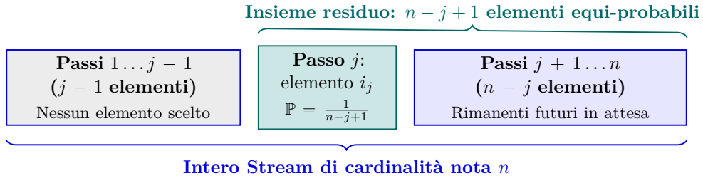
Figura 8.1: Partizione dello spazio dello stream al passo generico j per il campionamento a singolo elemento ( m = 1 ).
