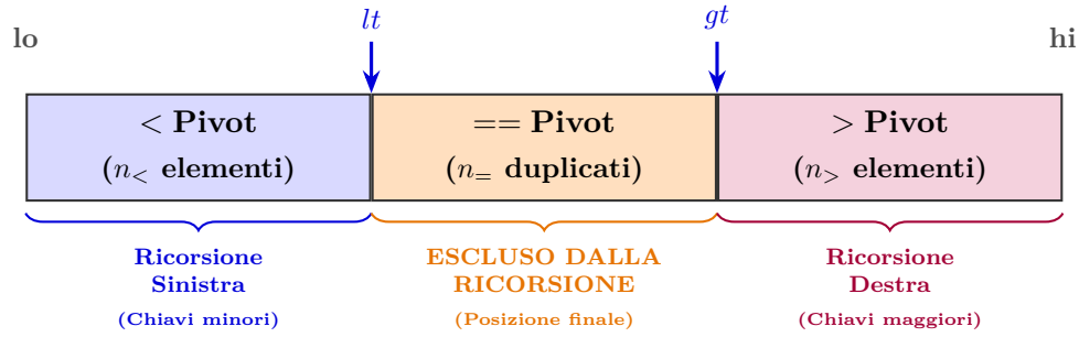
Figura 6.3: Topologia delle tre regioni del partizionamento a 3 vie ( Dutch National Flag ) e puntatori operativi lt e gt .
