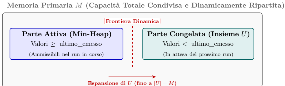
Figura 4.3: Ripartizione dinamica della memoria M durante la Replacement Selection (Spazzaneve).
