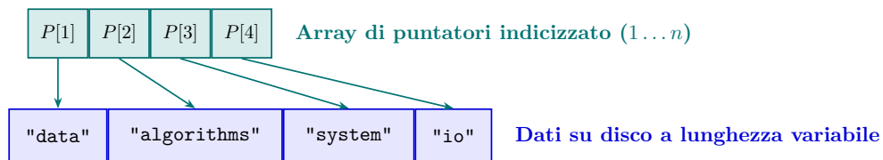
Figura 7.4: Mappatura di record a lunghezza variabile tramite array contiguo di puntatori indicizzato.
