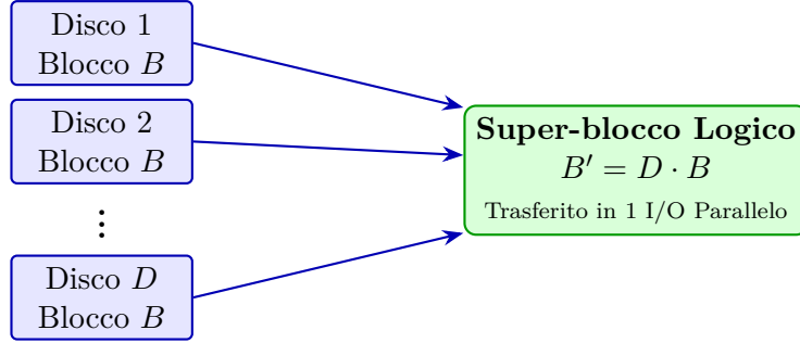
Figura 4.4: Architettura a Disk Striping: raggruppamento di D blocchi fisici in un super-blocco B' .
