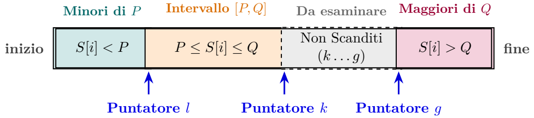
Figura 5.3: Schema del partizionamento nel Dual-Pivot Quicksort di Yaroslavskiy. L'array è partizionato nelle quattro regioni dinamiche: elementi < P , elementi compresi tra P e Q , elementi non ancora esaminati tra k e g , ed elementi > Q .
