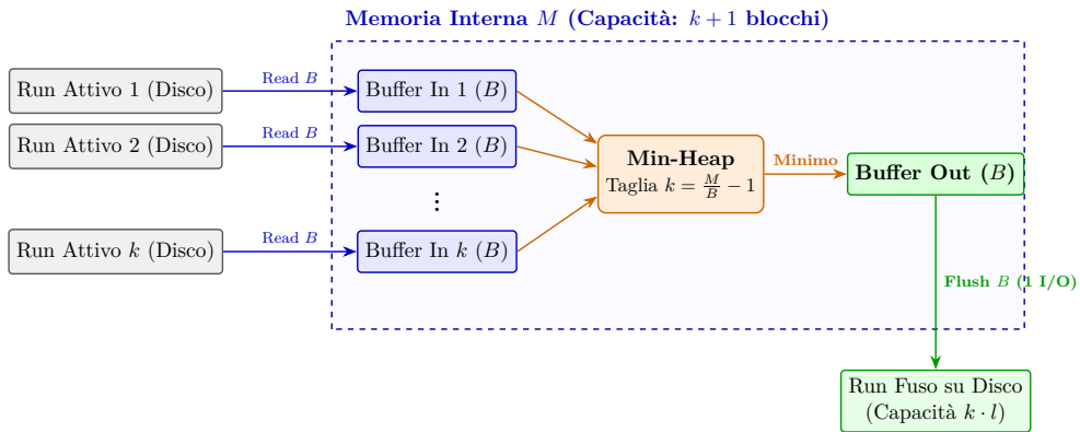
Figura 4.1: Architettura della memoria interna durante la fusione multi-via ( k -Way Merge Sort) con Min-Heap di coordinamento.
