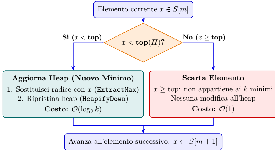
Figura 6.1: Flusso di elaborazione con Max-Heap di dimensione limitata k . Gli elementi che non migliorano i k minimi correnti vengono scartati in tempo costante \mathcal{O}(1) .
