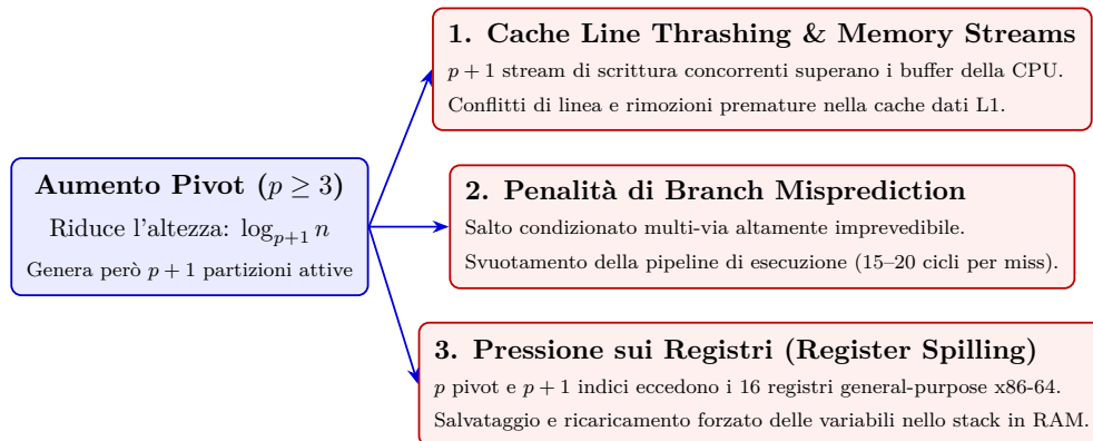
Figura 6.2: Cause microarchitetturali del decadimento prestazionale all'aumentare del numero di pivot p .
