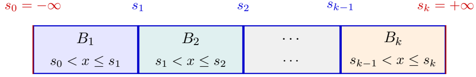
Figura 7.1: Partizionamento dell'insieme S in k secchielli ( buckets ) mediante k - 1 pivot ordinati.
