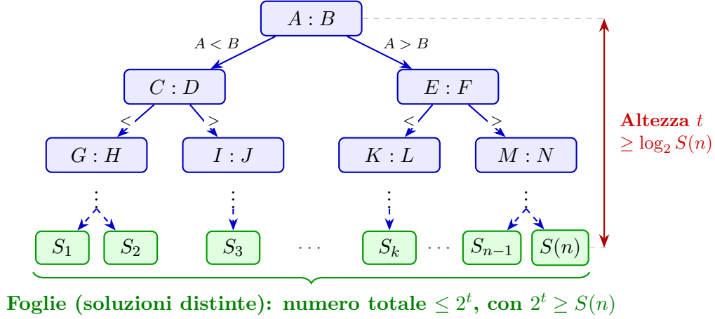
Figura 5.1: Modello dell'albero di decisione binario per algoritmi basati su confronti. I nodi interni rappresentano i confronti elementari; le foglie rappresentano le soluzioni distinte ammissibili ( S_1, S_2, \dots, S(n) ). Il cammino più lungo determina il tempo nel caso peggiore.
