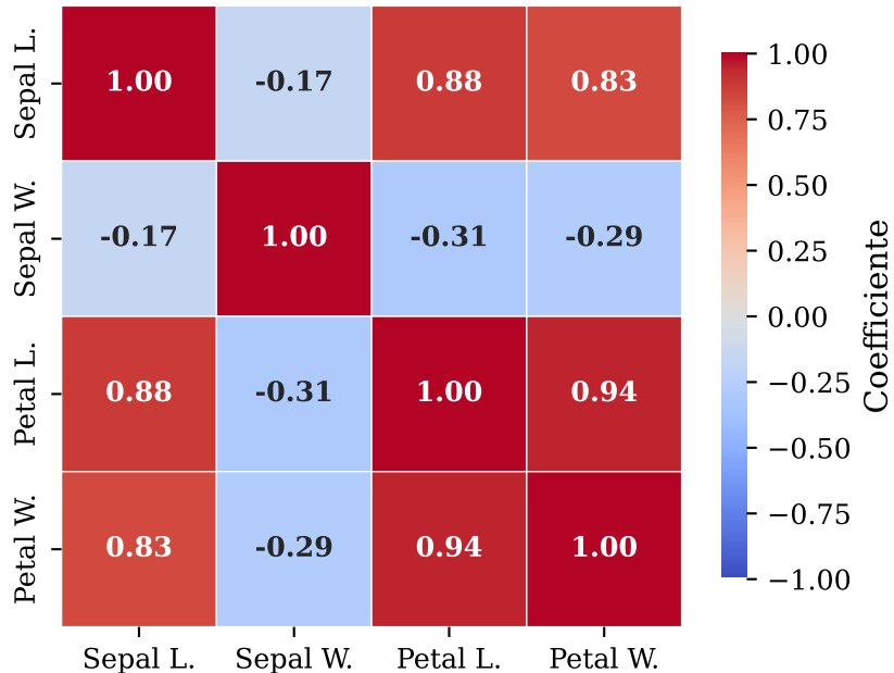
Correlazione di Rango di Spearman ( \rho_s )
