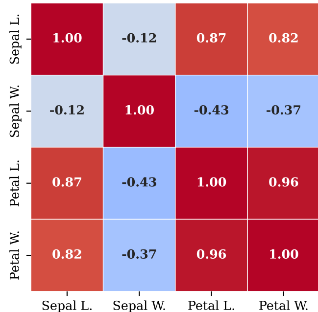
Correlazione Lineare di Pearson ( r )
