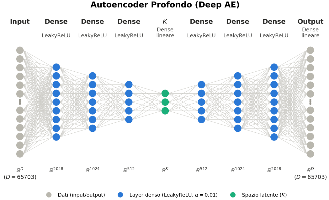
Figura 6.2. Architettura dell'Autoencoder Profondo (Deep AE): design a imbuto simmetrico con attivazione LeakyReLU sugli strati nascosti intermedi e nessuna attivazione sul layer di bottleneck e sull'ultimo layer del Decoder.
