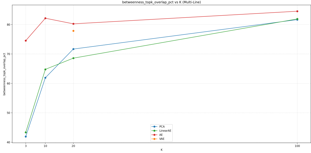
Figura 7.6. Percentuale di sovrapposizione fra i dieci nodi a più alta betweenness centrality dell'MST originale e quelli dell'MST ricostruito, dominio Cholesky, Test Set , in funzione di K . Valori più grandi corrispondono a una ricostruzione migliore ( \uparrow ).
