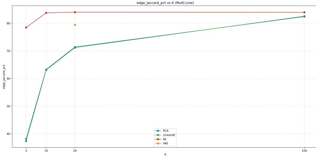
Figura 7.5. Indice di Jaccard fra l'insieme degli archi dell'MST della matrice originale e quello della matrice ricostruita, dominio Cholesky, Test Set , in funzione di K . Valori più grandi corrispondono a una ricostruzione migliore ( \uparrow ).
