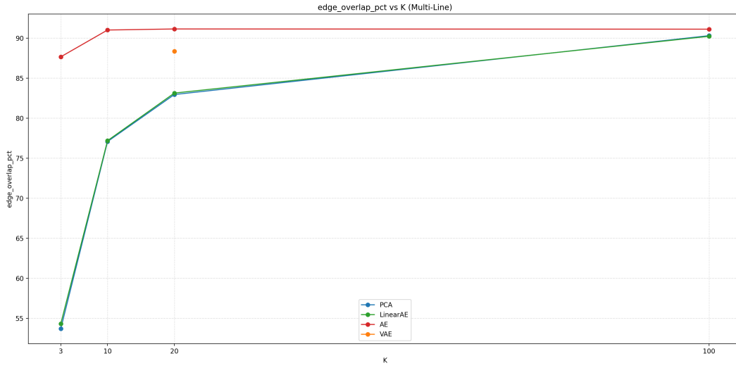
Figura 7.4. Percentuale di archi in comune tra l'MST della matrice originale e quello della matrice ricostruita, dominio Cholesky, Test Set , in funzione di K . Valori più grandi corrispondono a una ricostruzione migliore ( \uparrow ).
