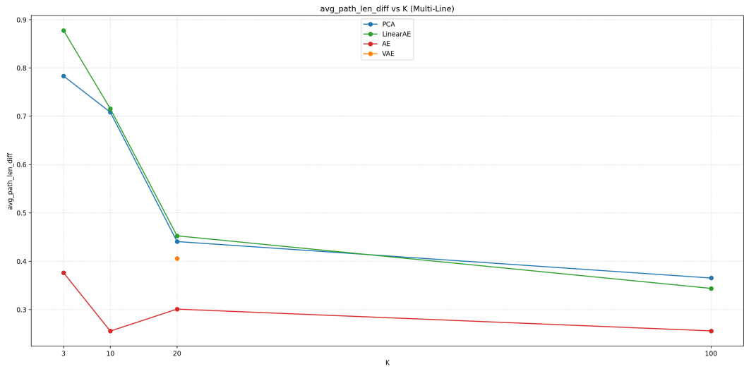
Figura 7.7. Scarto assoluto fra la lunghezza media dei cammini dell'MST originale e quella dell'MST ricostruito, versione pesata sulle distanze, dominio Cholesky, Test Set , in funzione di K . Trattandosi di uno scarto rispetto all'originale, qui il verso del confronto si inverte: valori più piccoli corrispondono a una ricostruzione migliore ( \downarrow ).
