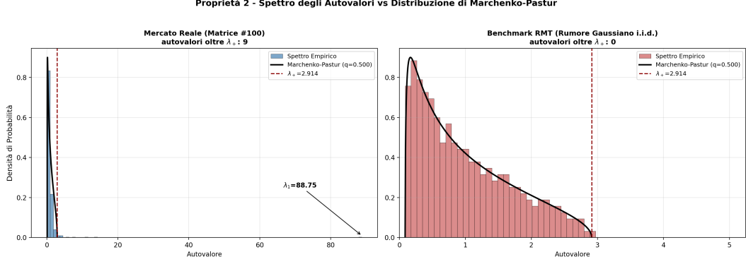
Figura 3.9. Proprietà 2 – Spettro degli autovalori contro la densità di Marchenko-Pastur ( q = 0.5 , \lambda_+ = 2.914 ): la matrice reale espone 9 autovalori oltre il bulk (incluso il modo di mercato \lambda_1 = 88.753 ), mentre il benchmark RMT non ne presenta alcuno ( \lambda_1 = 2.907 ).
