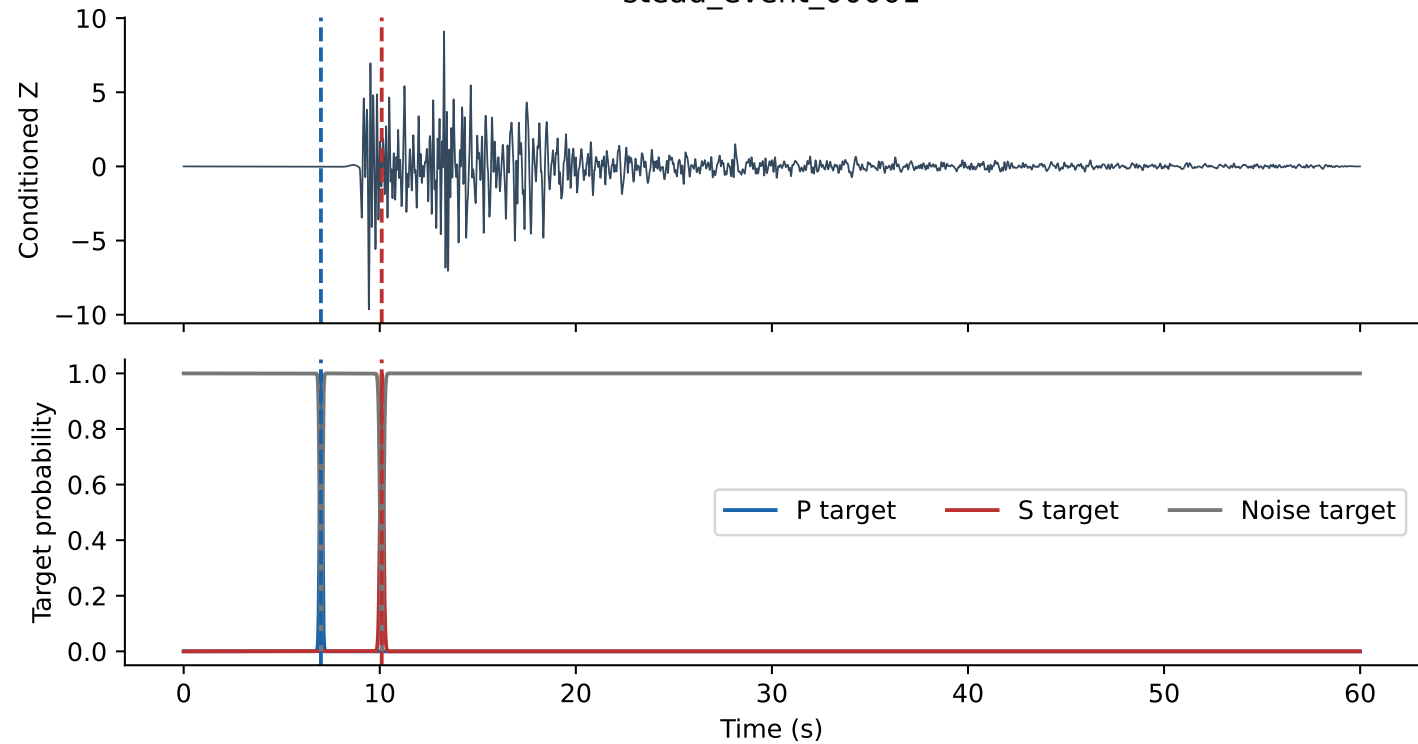
stead_event_00001
