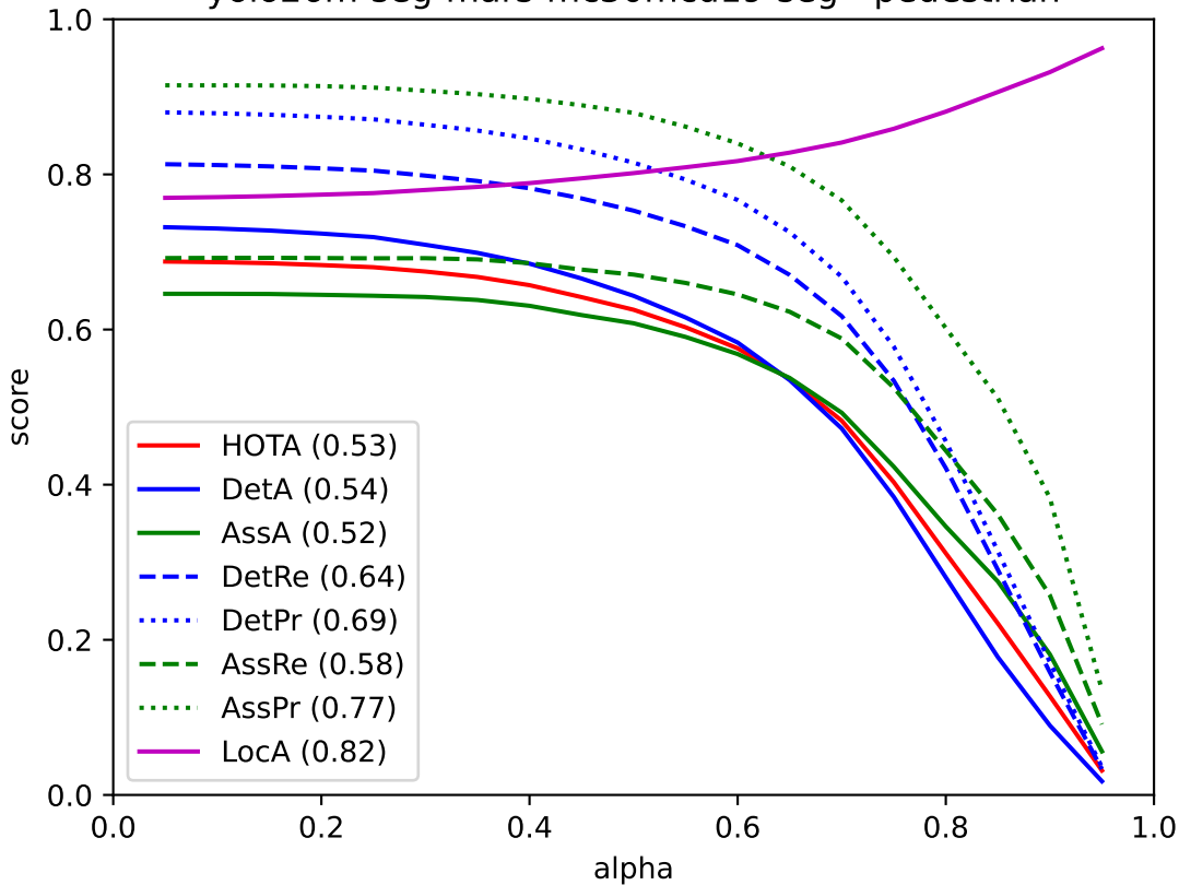
yolo26m-seg-mars-mc30mcd19-seg - pedestrian
