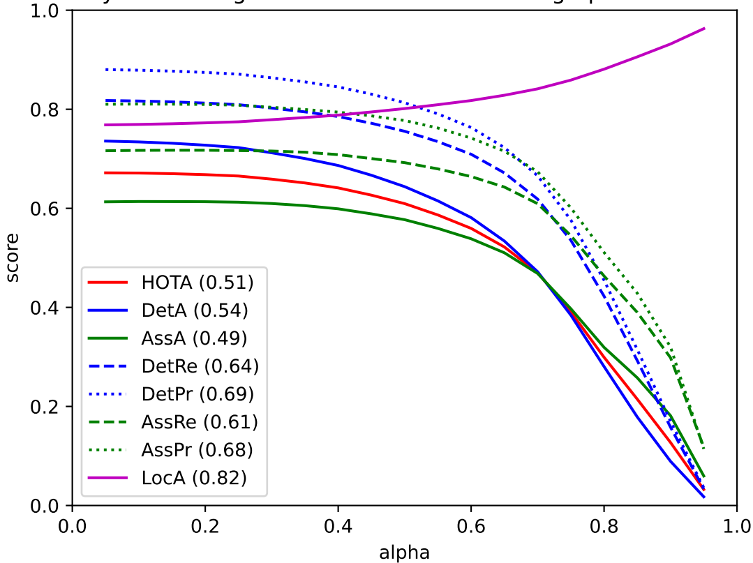
yolo26m-seg-mars-mc30mcd19mask-seg - pedestrian
