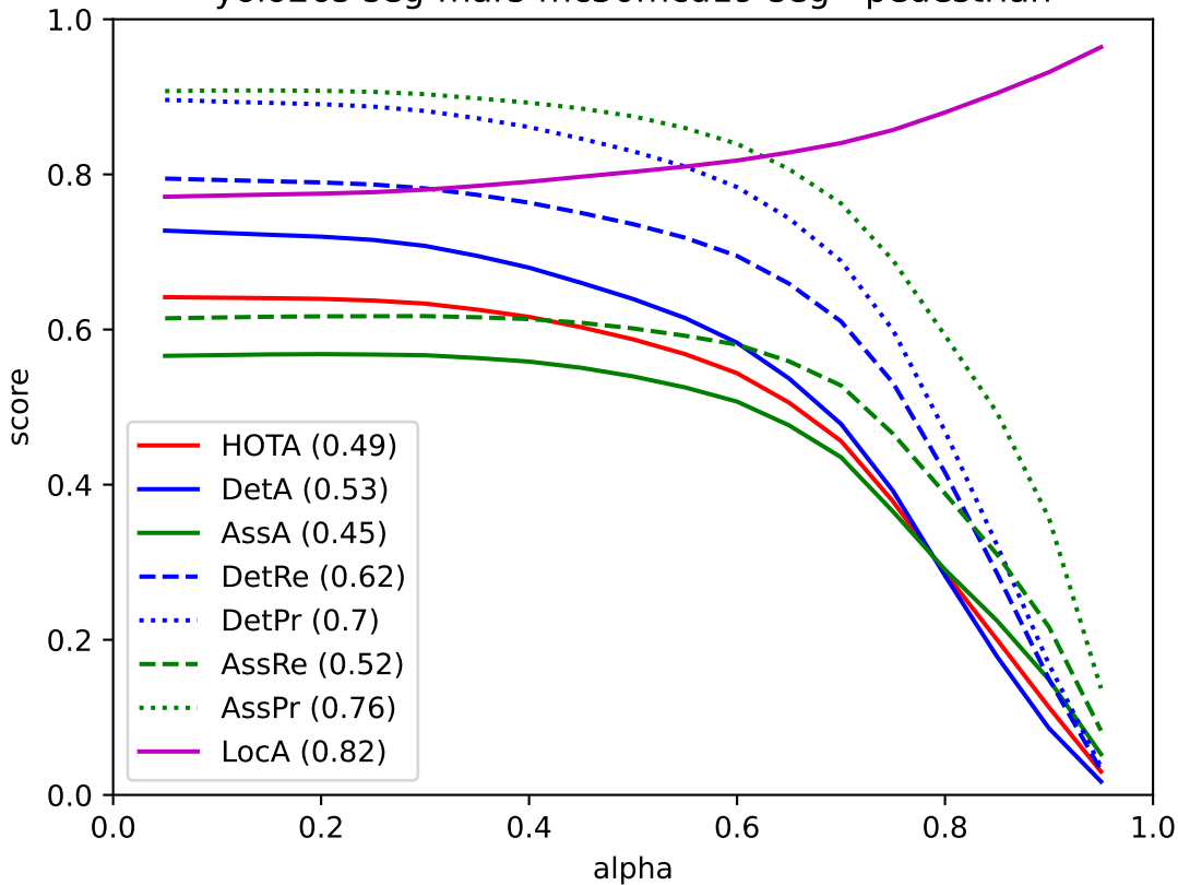
yolo26s-seg-mars-mc30mcd19-seg - pedestrian
