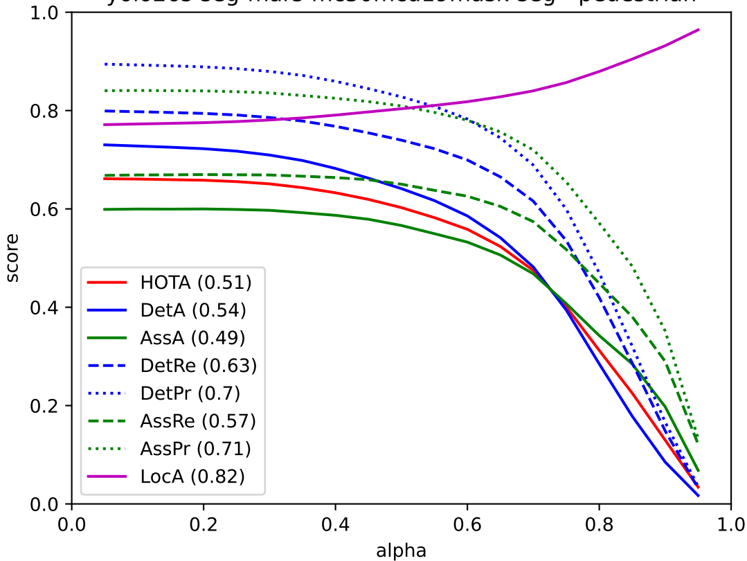
yolo26s-seg-mars-mc30mcd19mask-seg - pedestrian
