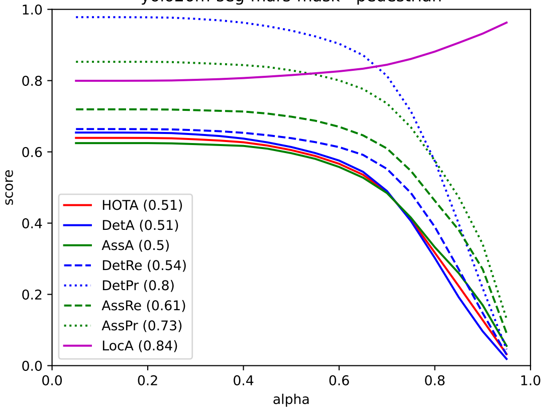
yolo26m-seg-mars-mask - pedestrian
