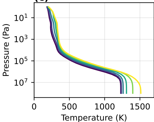
(c) \text{H}_2 + \text{H}_2\text{S}
