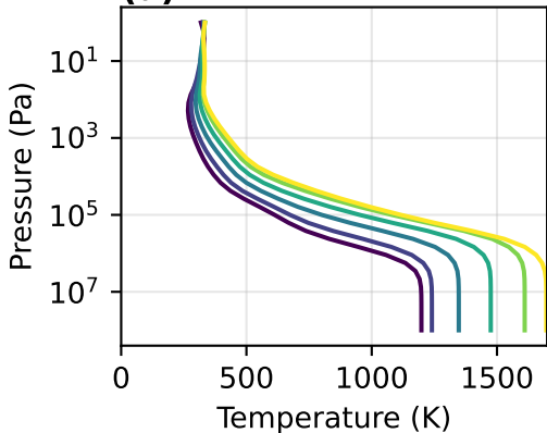
(a) \text{H}_2 + \text{H}_2\text{O}
