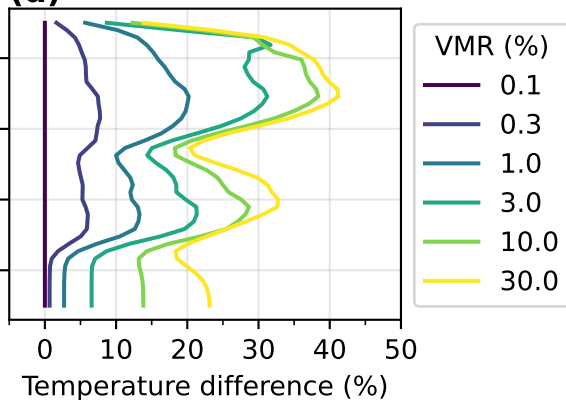
(d) \text{H}_2 + \text{H}_2\text{S}
