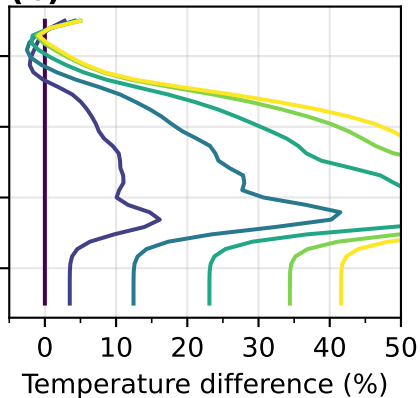
(b) \text{H}_2 + \text{H}_2\text{O}
