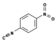
EVOSAJ
