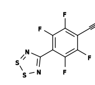
YOMXUT02
