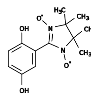
LICMIT01
