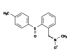
SANGIZ
