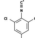
FUGVAE
