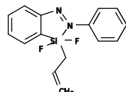
EZIPAE
