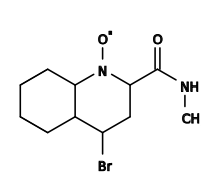
MULNIR
