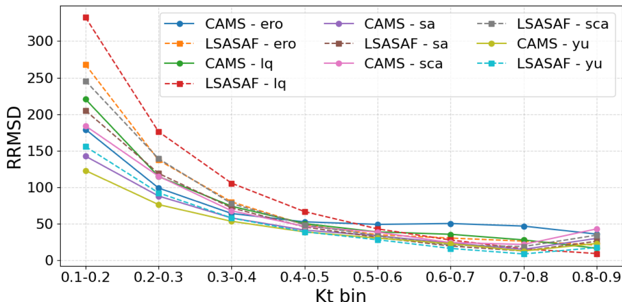
Figura 3.4: Variación del error cuadrático medio relativo (RRMSD) en función del índice de claridad ( k_t ) para los cinco sitios analizados (YU, SA, SCA, ERO y LQ). Resultados para CAMS (líneas continuas) y LSASAF (líneas punteadas).
