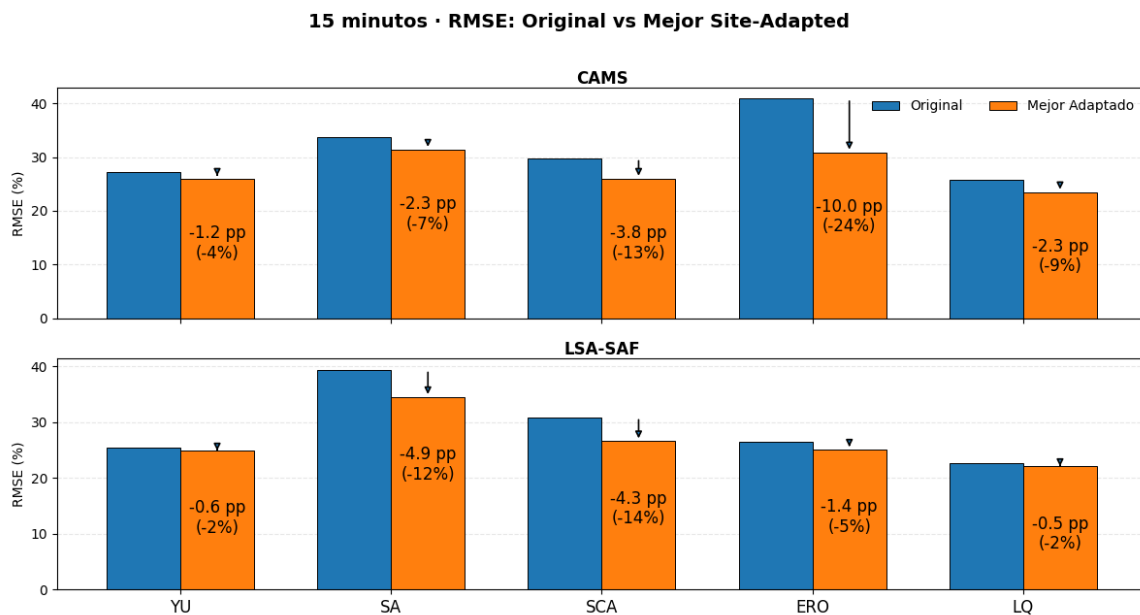
Figura 3.15: Comparación del RMSE(%) para los modelos crudos y el mejor desempeño obtenido.
