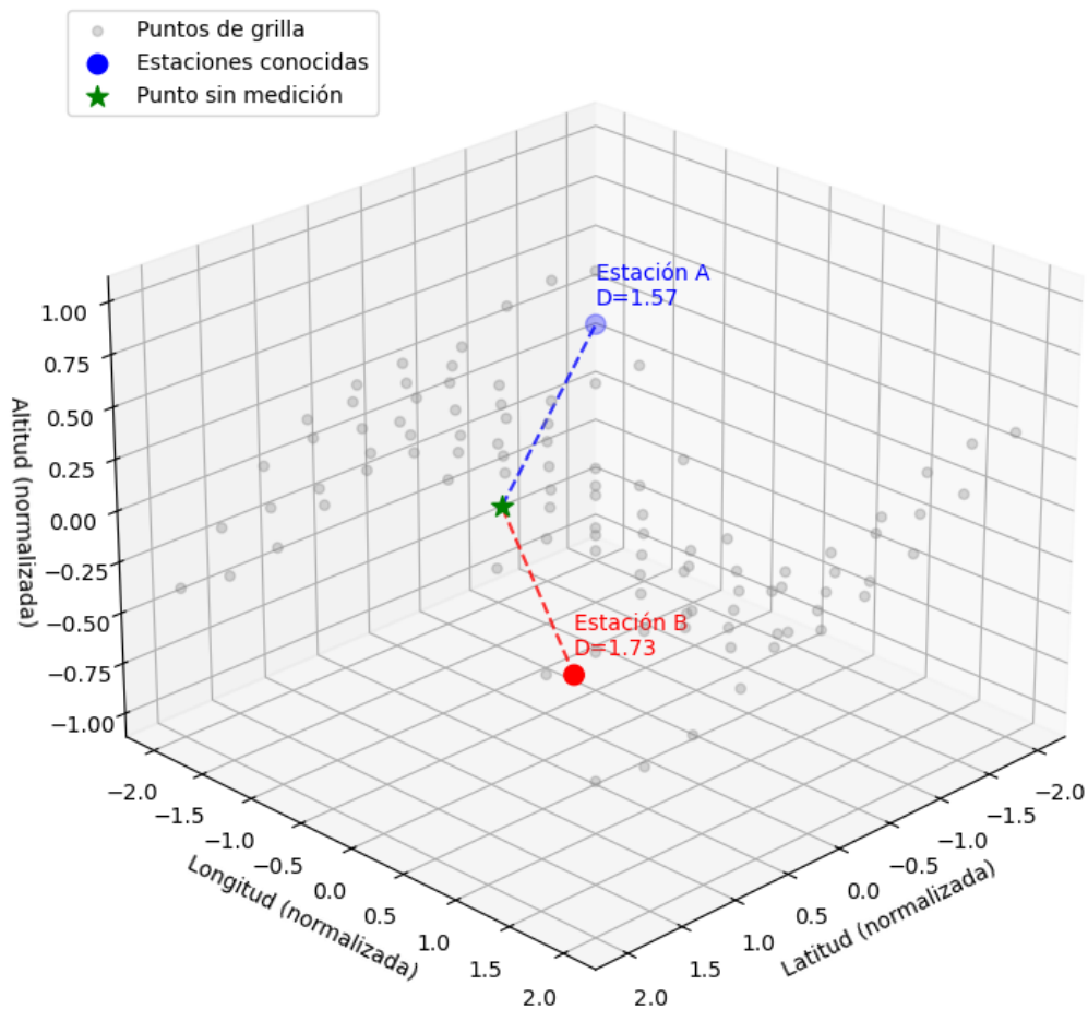
Figura 3.27: Ejemplo de asignación por distancia geográfica y altitudinal (normalizada). En gris se representan los puntos donde se pretende aplicar la generalización (sin medición). Los puntos azul y rojo indican estaciones A y B (con medición directa). En verde se muestra el punto objetivo sin medición, que recibe el modelo de la estación más cercana. Las líneas punteadas indican las distancias tridimensionales calculadas tras la normalización, señalando cuál de ellas es menor (la que define el modelo asignado).
