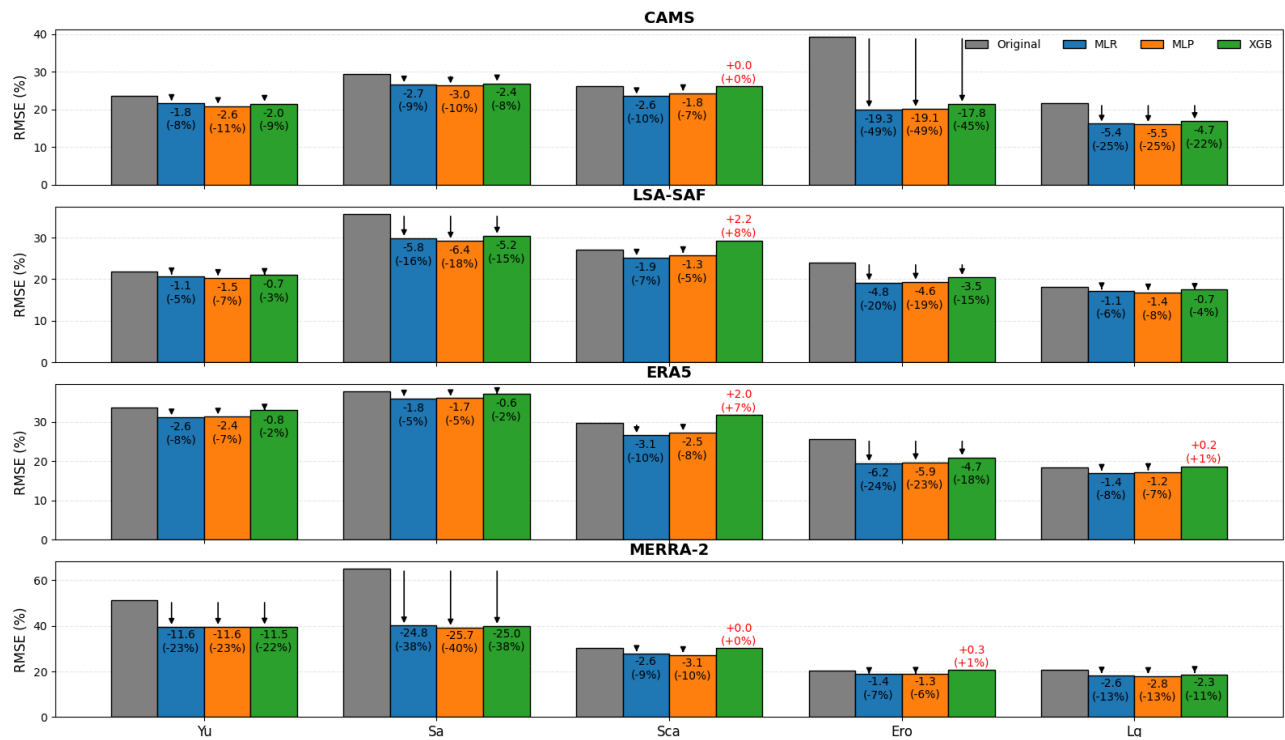
Figura 3.17: Comparación del rRMSE% entre estimaciones originales de los satélites y sus versiones adaptadas mediante los regresores MLR, MLP y XGB para los cinco sitios (Yu, Sa, Sca, Ero y Lq). Las flechas indican mejora en la métrica adaptada respecto al valor original; las anotaciones muestran el cambio absoluto y relativo. Las flechas negras representan mejoras, mientras que las flechas rojas indican empeoramiento del desempeño respecto al modelo original.
