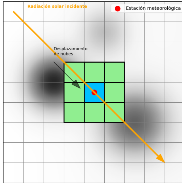
Figura 3.21: Analogía espacial: celdas del producto de GHI y dinámica atmosférica
