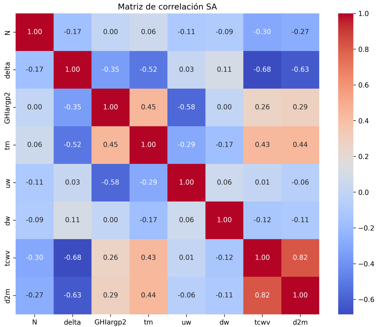
Figura 3.19: Coeficientes de correlación de Pearson y Spearman entre las variables meteorológicas y las distintas metodologías (Yu, Sa, Sca, Ero y Lq).
