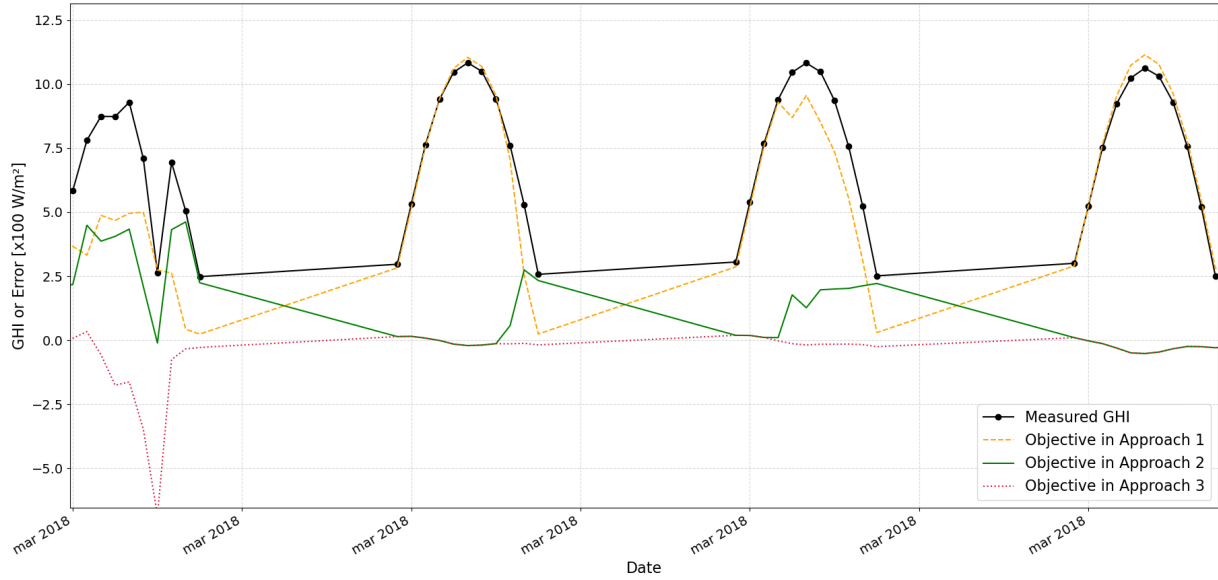
Figura 3.24: Diferencias entre los tres enfoques de adaptación.
