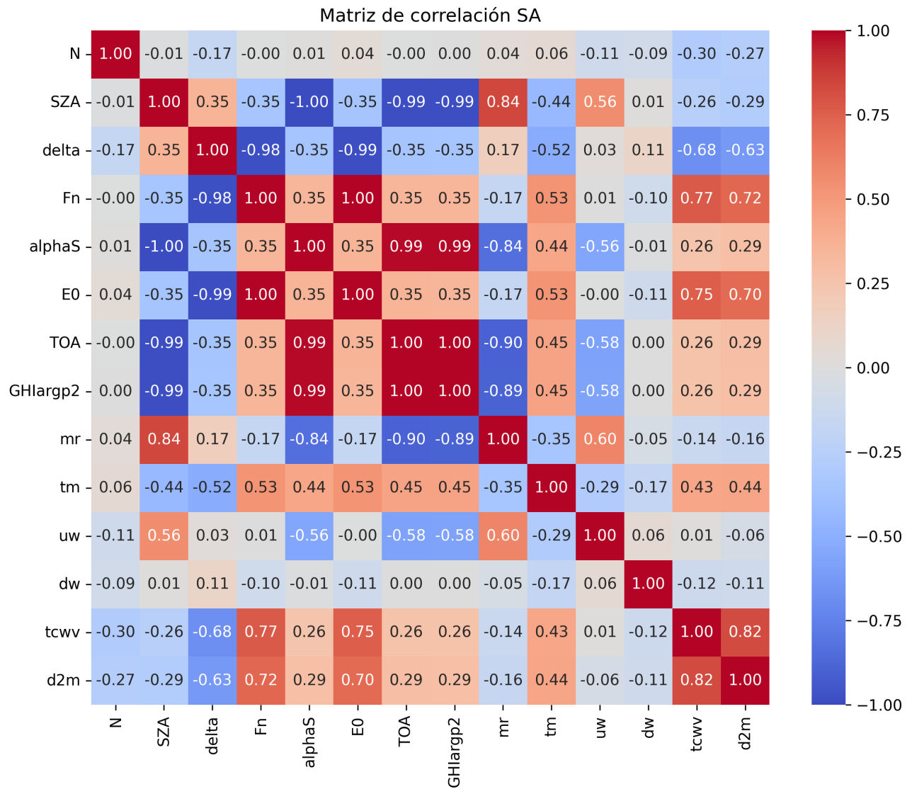
Figura 3.18: Matriz de correlación de los regresores en la estación SA.
