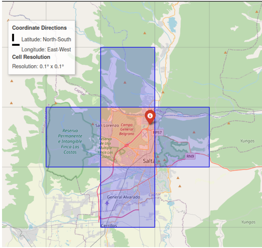
Figura 3.22: Grilla utilizada por el modelo Helisat-4 de CAMS distribuido por CAMS Volume
