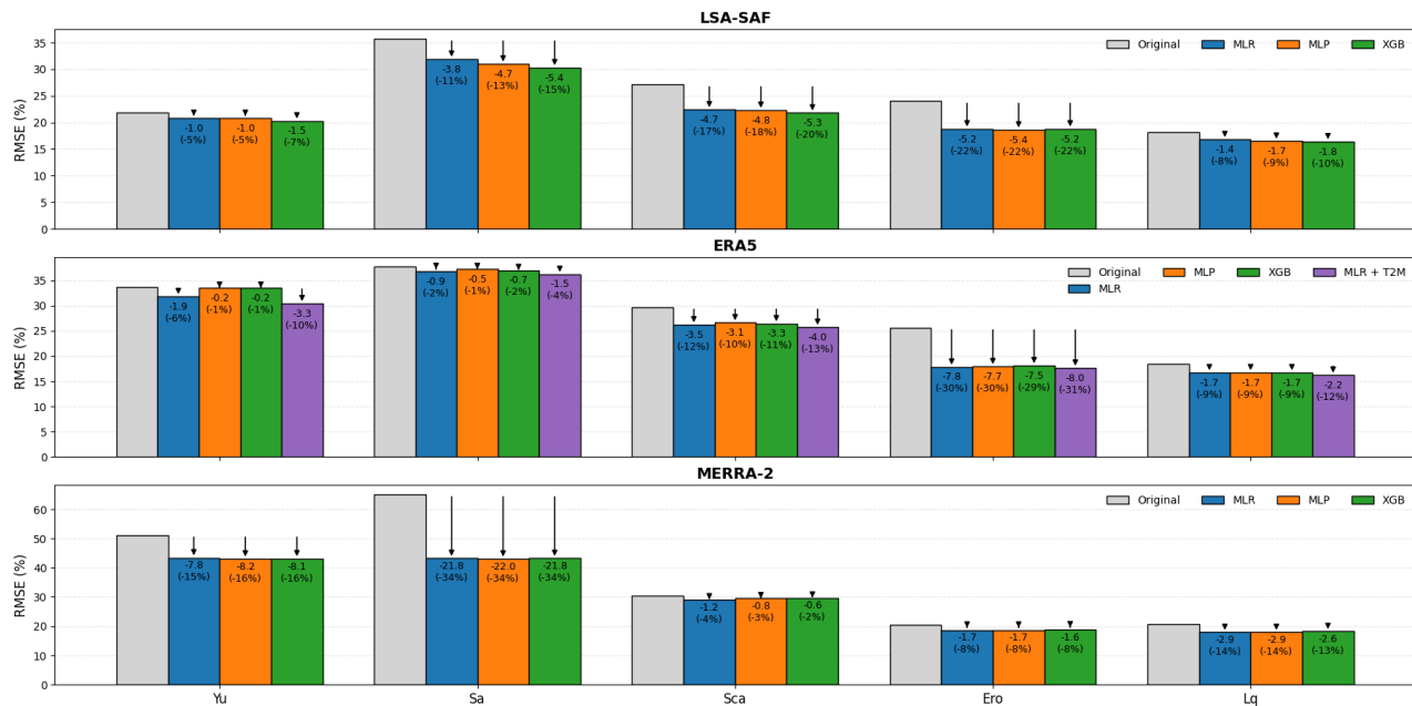
Figura 3.23: RMSD(%) comparativo para las evaluaciones utilizando el enfoque de celdas adyacentes
