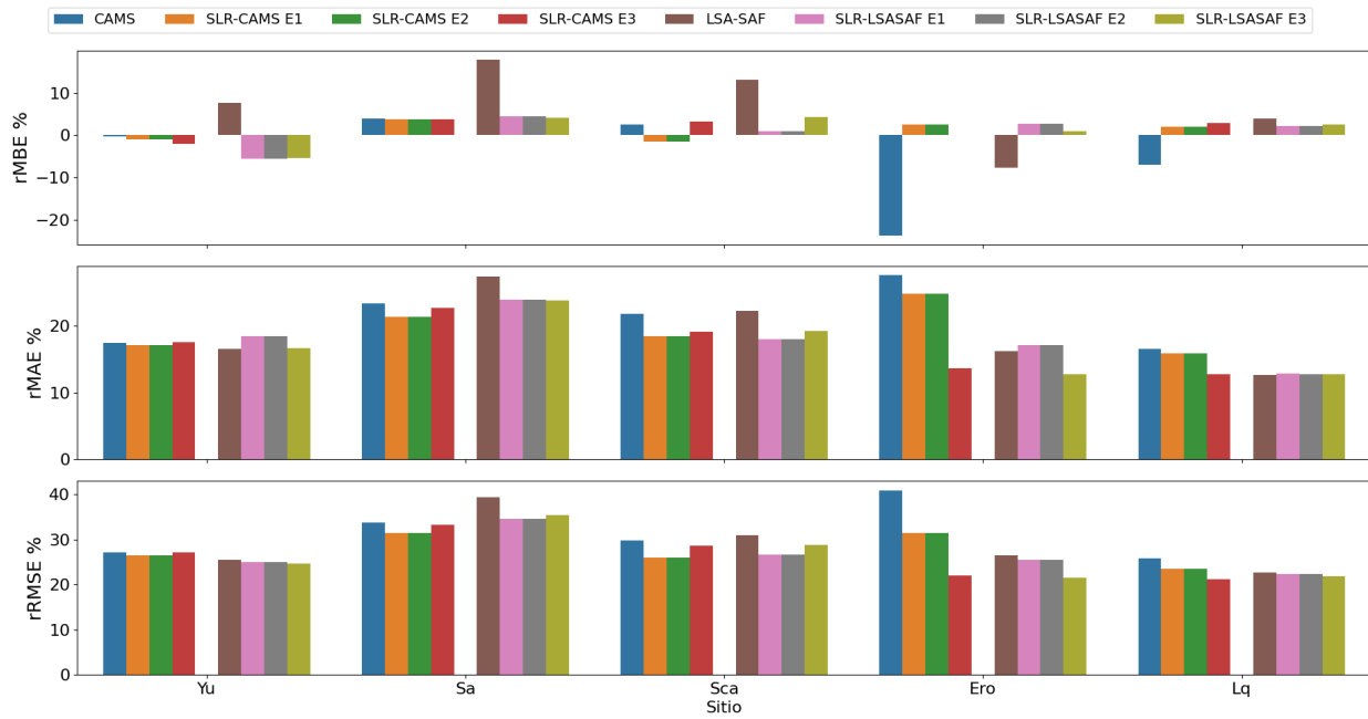
Figura 3.23: Métricas de desempeño relativas ( rMBE , rMAE y rRMSE , en %) obtenidas en los cinco sitios de prueba (Yu, Sa, Sca, Ero y Lq). Se comparan las estimaciones satelitales originales (CAMS y LSA-SAF) con sus adaptaciones al sitio mediante los enfoques E1, E2 y E3. En cada subplot se agrupan las barras por sitio, mostrando primero los modelos basados en CAMS y luego, separados visualmente, los modelos basados en LSA-SAF.
