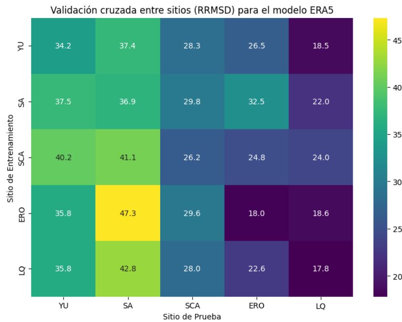
Figura 3.20: Matriz de rRMSD (%) obtenida a partir de la validación cruzada entre sitios para el modelo ERA5, utilizando los modelos ajustados con celdas satelitales adyacentes al sitio de interés.
