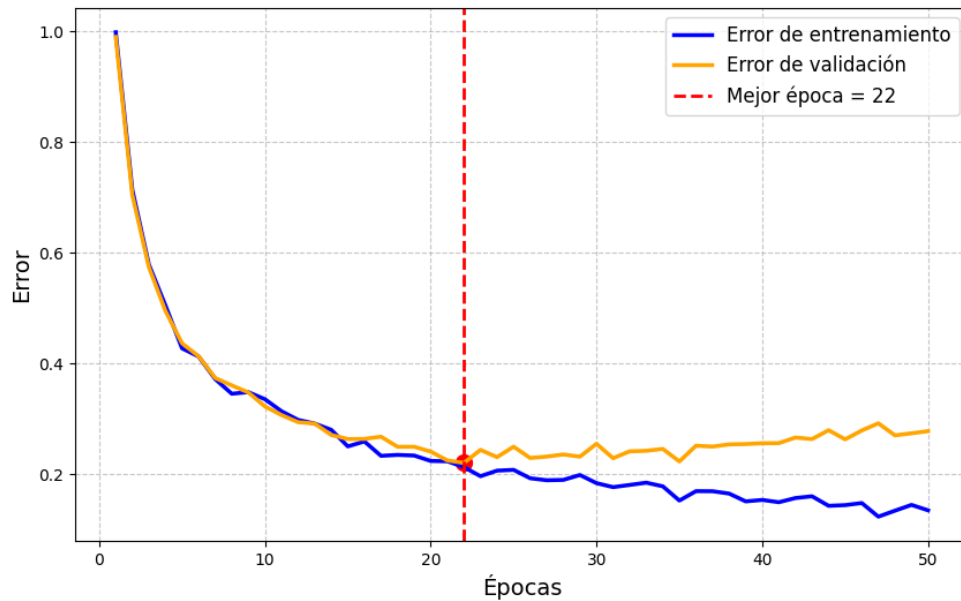
Figura 2.6: Dinámica de entrenamiento de un modelo de aprendizaje automático. La curva azul muestra el error de entrenamiento, que disminuye progresivamente a medida que el modelo se ajusta a los datos. La curva naranja representa el error de validación, que disminuye inicialmente reflejando la mejora de la capacidad de generalización, pero comienza a aumentar después de la mejor época (línea roja discontinua), evidenciando el sobreajuste.
