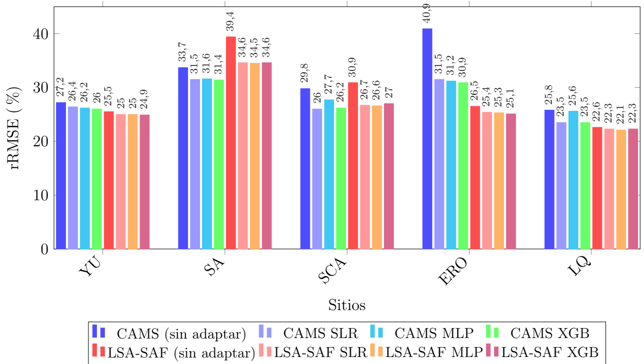
Figura 3.9: rRMSE(%) ( en resolución de 15 minutos para cada modelo y sitio, comparando modelos sin adaptación y adaptados.
