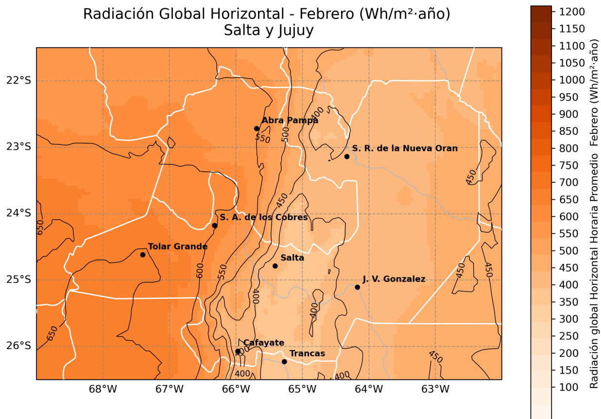
Figura 4.2: Mapa de GHI medio mensual – Febrero (TMY).
