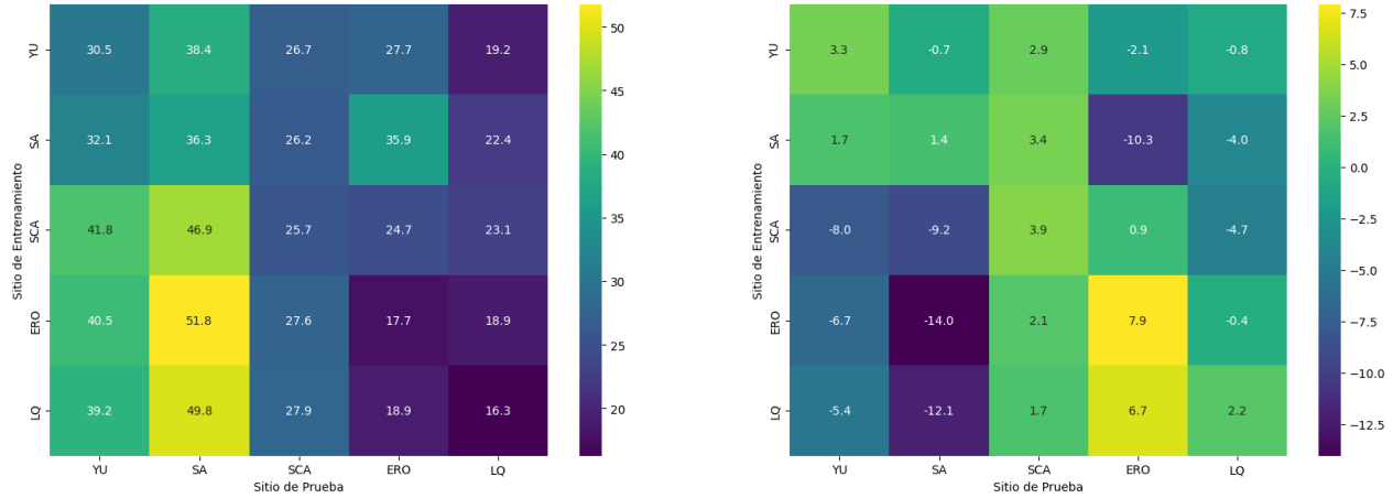
(a) Matriz de rRMSE (%) obtenida a partir de la validación cruzada entre sitios para el modelo ERA5, utilizando los modelos ajustados con celdas satelitales adyacentes al sitio de interés.
