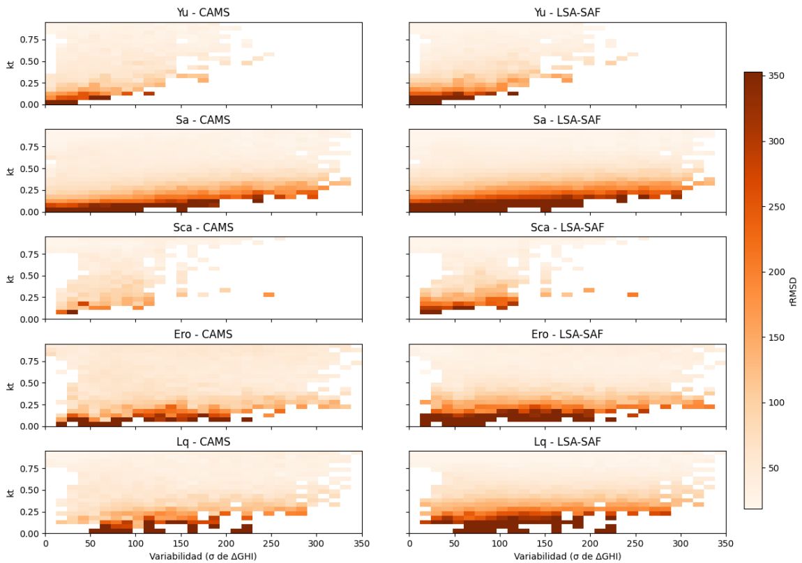
Figura 3.4: Distribución del error relativo cuadrático medio ( rRMSE ) en función del índice de claridad ( k_t ) y un índice de variabilidad calculado a partir de la desviación estándar de las diferencias consecutivas de GHI.
