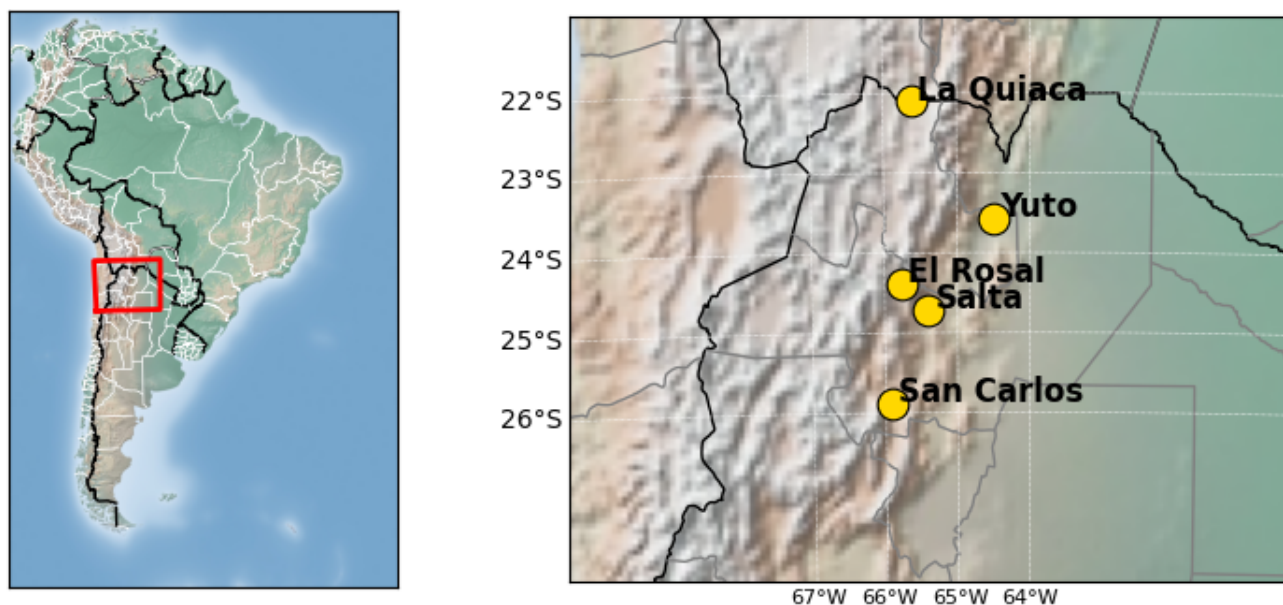
Figura 3.1: Ubicación de la estaciones de medida
