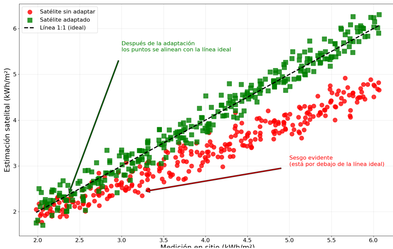
Figura 2.2: Diagrama de dispersión entre mediciones en sitio y estimaciones satelitales. Antes de la adaptación (puntos rojos), los datos muestran un sesgo claro al situarse por debajo de la línea 1:1. Después de la adaptación (puntos verdes), las estimaciones se alinean mucho mejor con la referencia, reduciendo el error sistemático.
