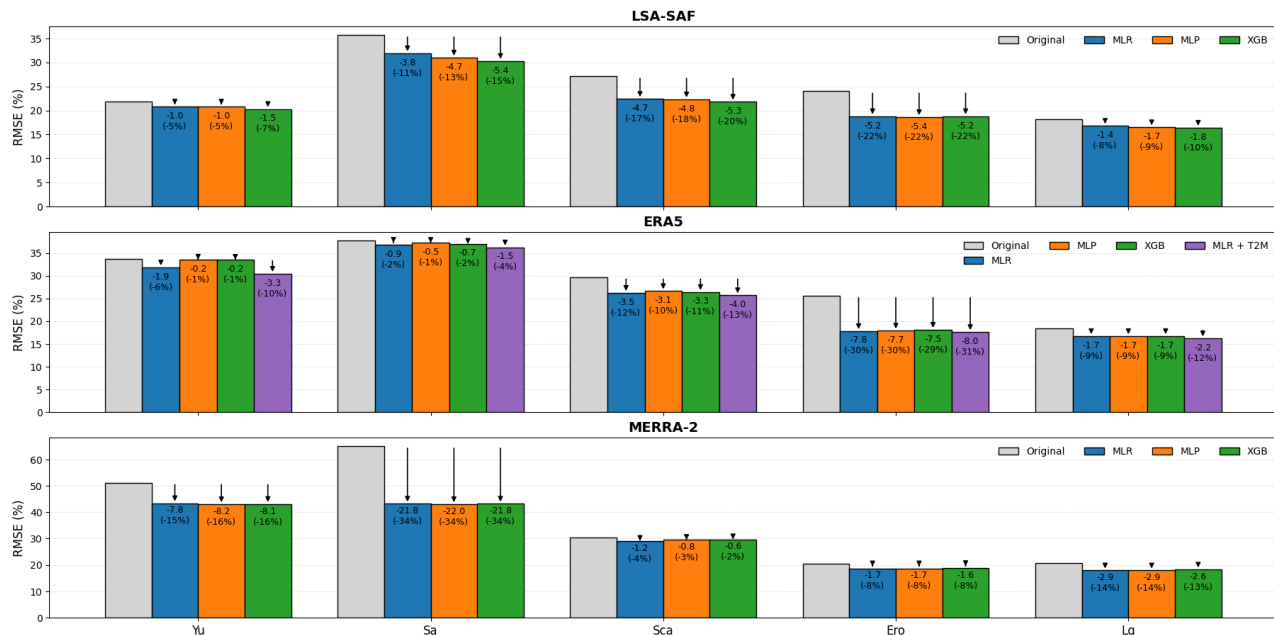
Figura 3.23: rRMSE(%) comparativo para las evaluaciones utilizando el enfoque de celdas adyacentes
