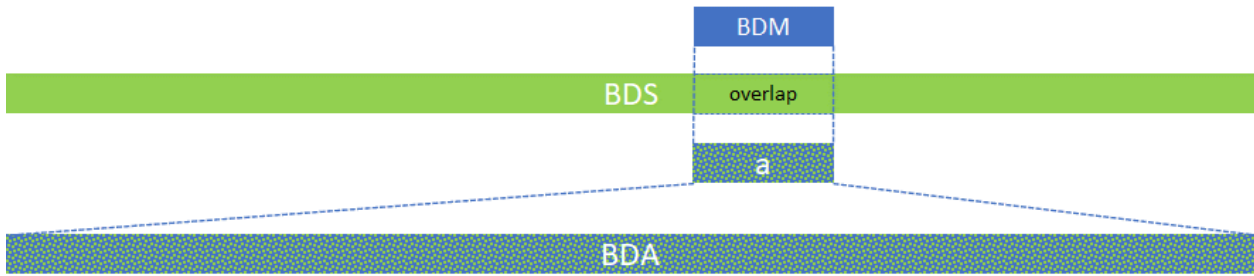
Figura 2.1: Esquema conceptual del proceso de adaptación al sitio.
