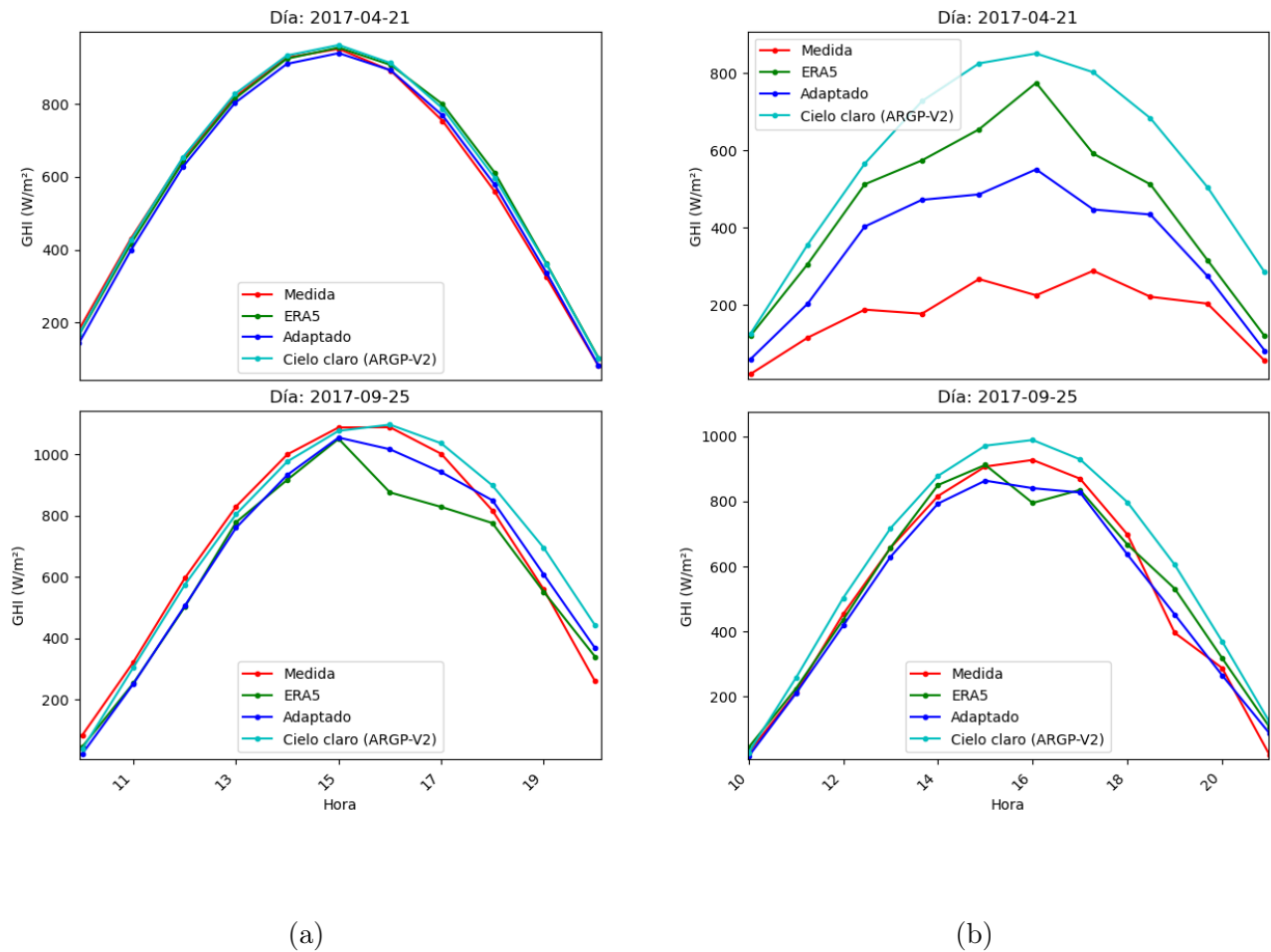
Figura 3.28: Comparación entre la GHI medida y la estimada mediante el criterio de generalización propuesto para el reanálisis ERA5 en los sitios de Abra Pampa (a) y Cerrillos (b).
