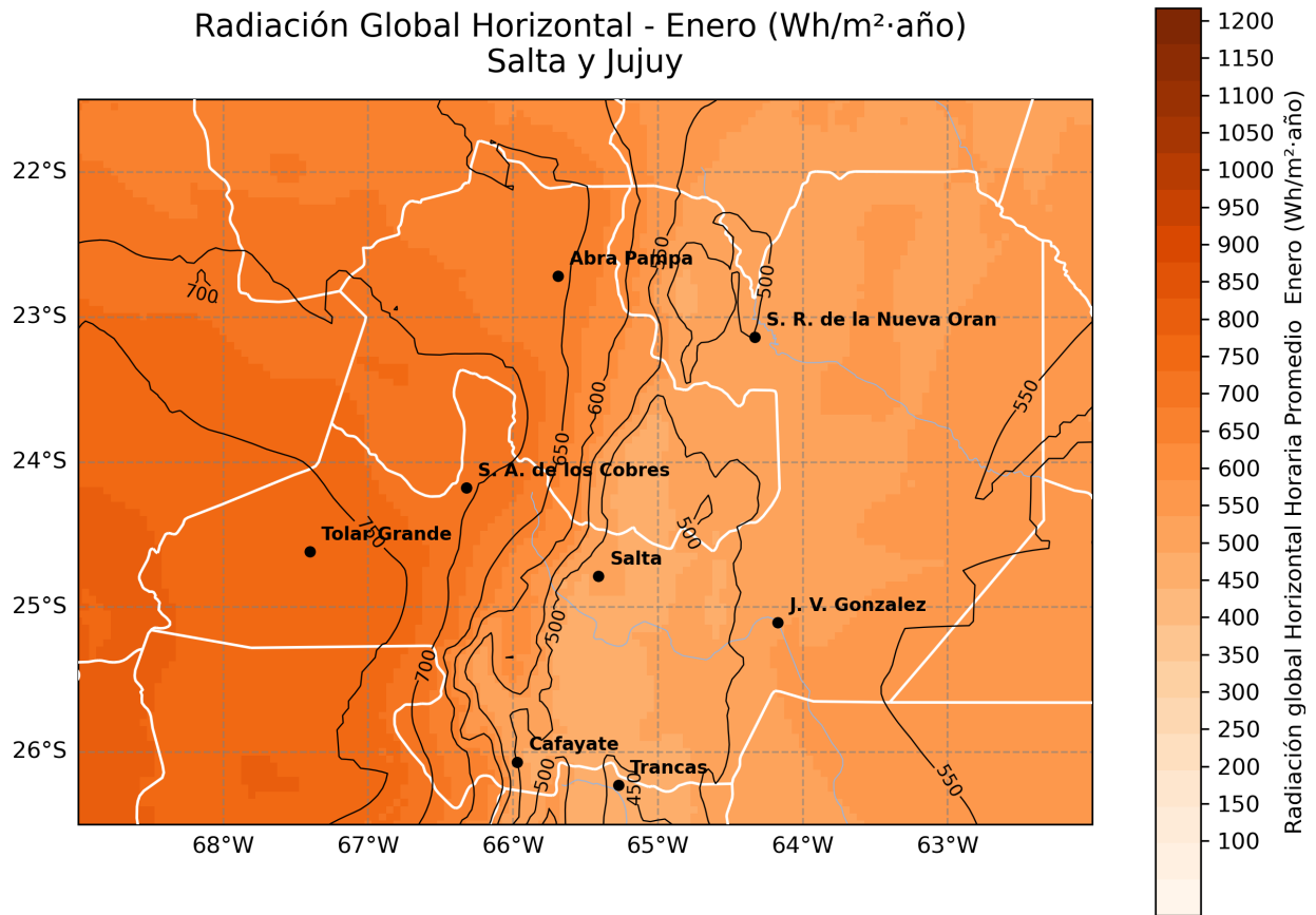
Figura 4.1: Mapa de GHI medio mensual – Enero (TMY).
