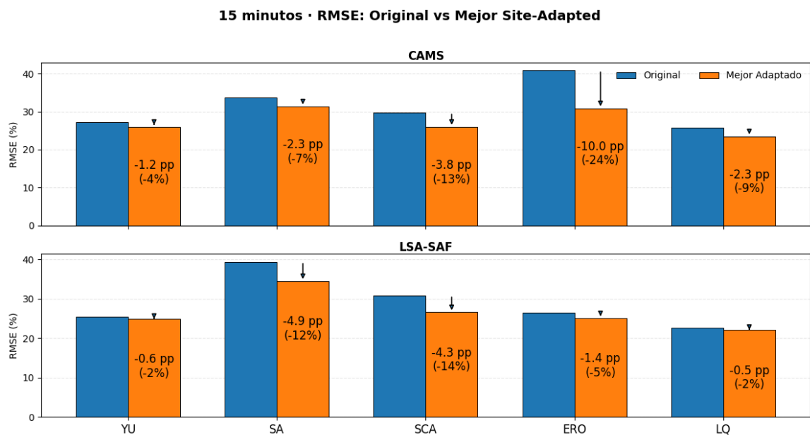
Figura 3.15: Comparación del rRMSE(%) para los modelos crudos y el mejor desempeño obtenido.
