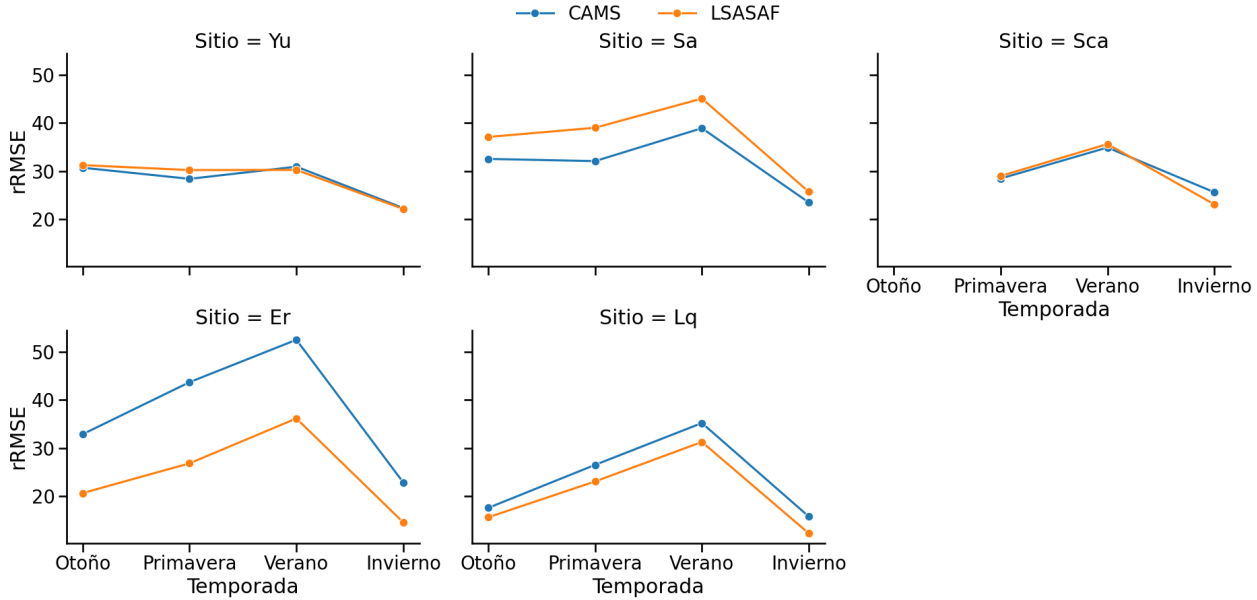
Figura 3.3: Variación estacional del rRMSE (%) para los productos CAMS y LSA-SAF con resolución de 15 minutos en todos los sitios de estudio. Se evidencia un aumento del error durante el verano en la mayoría de los sitios, mientras que en Yuto el rRMSE se mantiene estable, sugiriendo que la presencia de nubosidad estacional afecta de manera diferenciada la precisión de las estimaciones de radiación solar.
