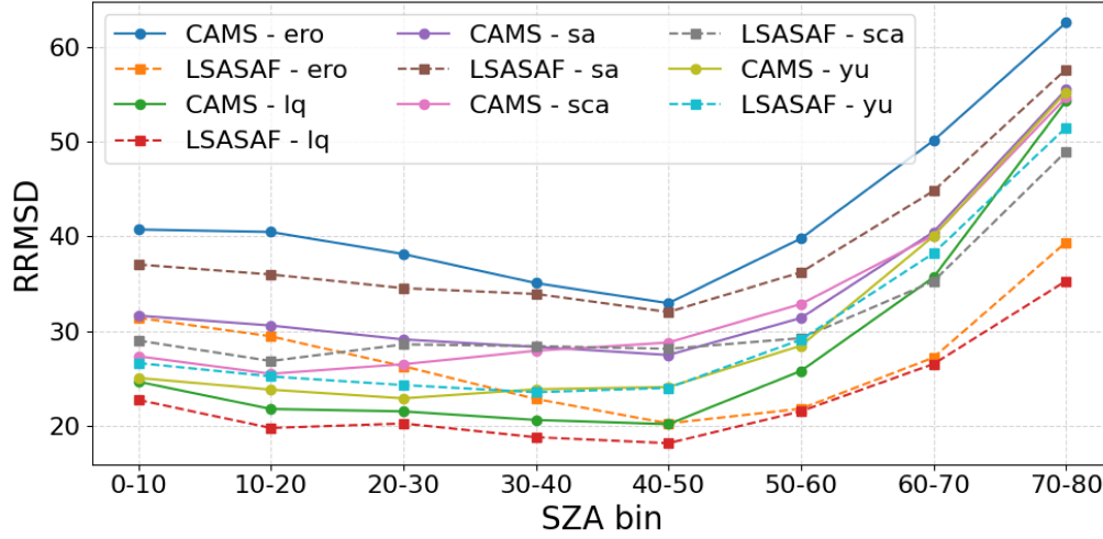
Figura 3.5: Variación del error cuadrático medio relativo ( rRMSE ) en función del ángulo cenital solar (SZA) para los cinco sitios analizados (Yu, Sa, Sca, Ero y Lq). Resultados para CAMS (líneas continuas) y LSA-SAF (líneas punteadas).
