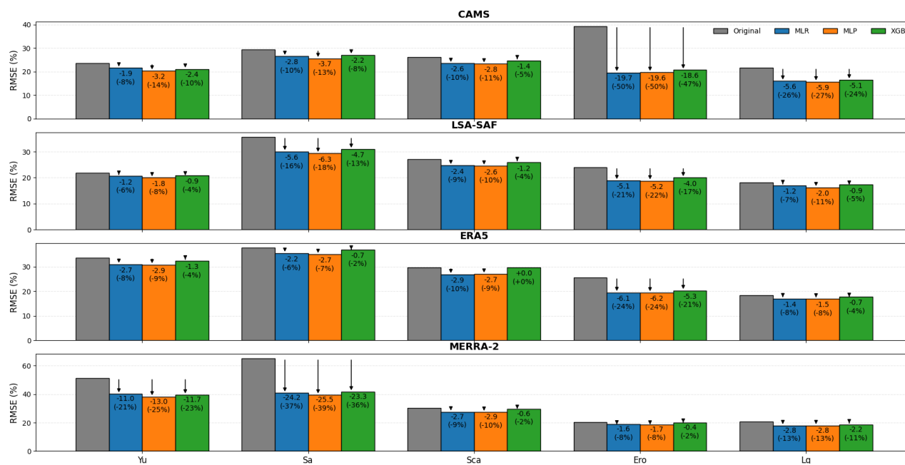
Figura 3.20: Comparación del rRMSE% entre estimaciones originales de los satélites y sus versiones adaptadas mediante los regresores MLR, MLP y XGB para los cinco sitios (Yu, Sa, Sca, Ero y Lq) utilizando como regresores la GHI estimada por cada modelo, GHIargp2 y tm. Las flechas indican mejora en la métrica adaptada respecto al valor original; las anotaciones muestran el cambio absoluto y relativo. Las flechas negras representan mejoras, mientras que las flechas rojas indican empeoramiento del desempeño respecto al modelo original.
