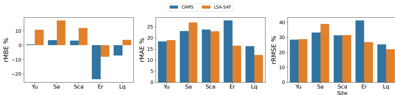
Figura 3.2: Comparación del desempeño de los modelos CAMS y LSA-SAF en los cinco sitios de estudio (Yu, Sa, Sca, Er y Lq) mediante las tres métricas estadísticas: MBE, MAE y RMSE expresadas en términos porcentuales relativos a escala 15-minutal.
