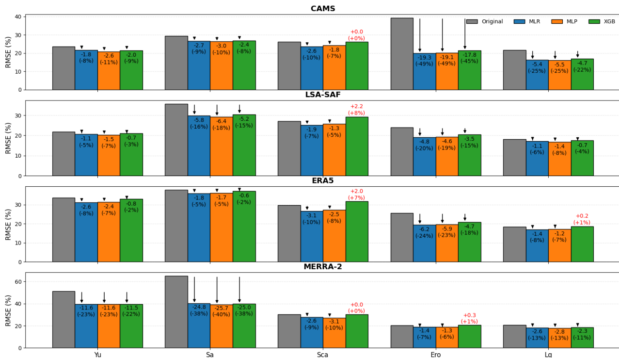
Figura 3.17: Comparación del rRMSE % entre estimaciones originales de los satélites y sus versiones adaptadas mediante los regresores MLR, MLP y XGB para los cinco sitios (Yu, Sa, Sca, Ero y Lq). Las flechas indican mejora en la métrica adaptada respecto al valor original; las anotaciones muestran el cambio absoluto y relativo. Las flechas negras representan mejoras, mientras que las flechas rojas indican empeoramiento del desempeño respecto al modelo original.
