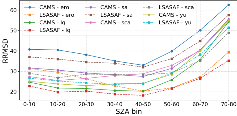
Figura 3.5: Variación del error cuadrático medio relativo (rRMSE) en función del ángulo cenital solar (SZA) para los cinco sitios analizados (Yu, Sa, Sca, Ero y Lq). Resultados para CAMS (líneas continuas) y LSA-SAF (líneas punteadas).
