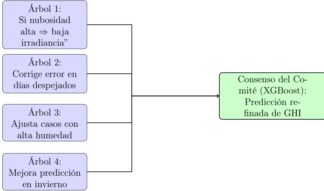
Figura 2.10: Analogía del comité de expertos en XGBoost: cada árbol corrige los errores de sus predecesores y contribuye a una predicción final más precisa de la GHI.
