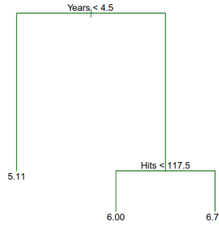
Figura 2.9: Ejemplo Árbol de Regresión. Para los datos de Hitters, se construye un árbol de regresión para predecir el logaritmo del salario de un jugador de béisbol, en función del número de años que ha jugado en las grandes ligas y el número de hits que realizó en el año anterior.
